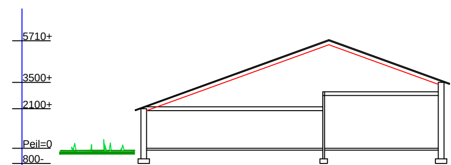
DOORSNEDE A-A , gebouw 2
