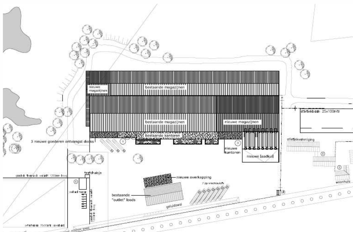
Figuur 3.1. De voorgestane situatie. Bron: Van Beijsterveldt & Gommers Architecten.
