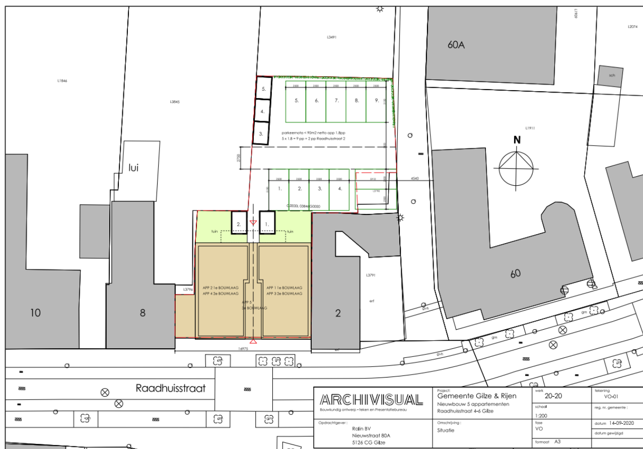
Figuur 3.1. Schets van de voorgestane situatie. Bron: Archivisual
