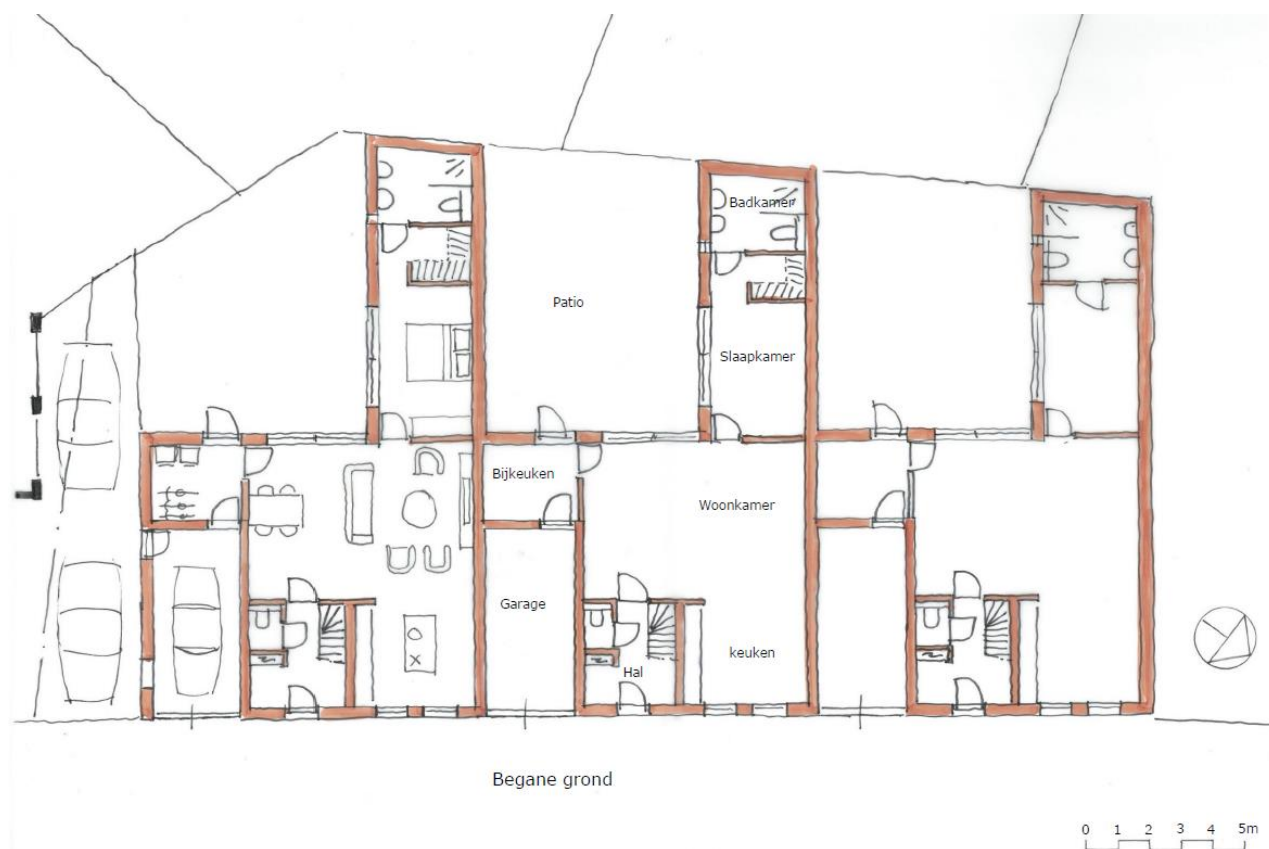
Figuur 3.1. De voorgestane situatie. In het plangebied worden drie patiowoningen gerealiseerd. Bron: Van Beijsterveldt & Gommers Architecten.
