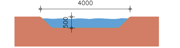
Doorsnede sloot
