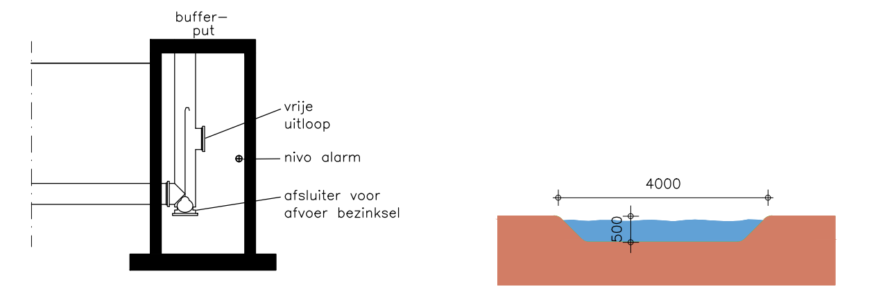
Doorsnede bufferput
