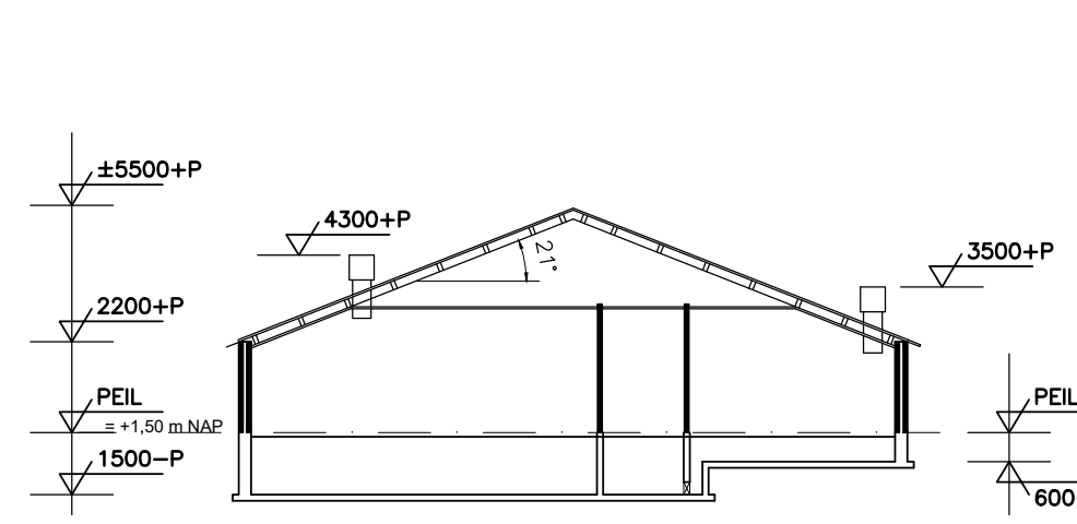
Doorsnede B-B
