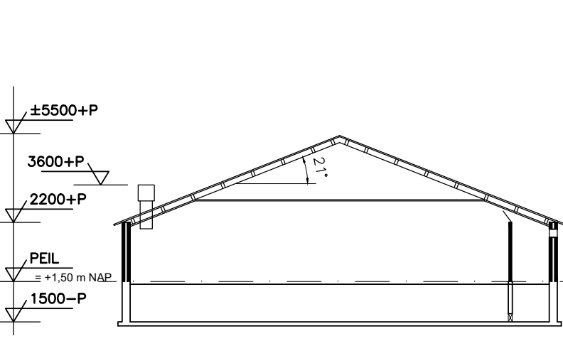
Doorsnede D-D
