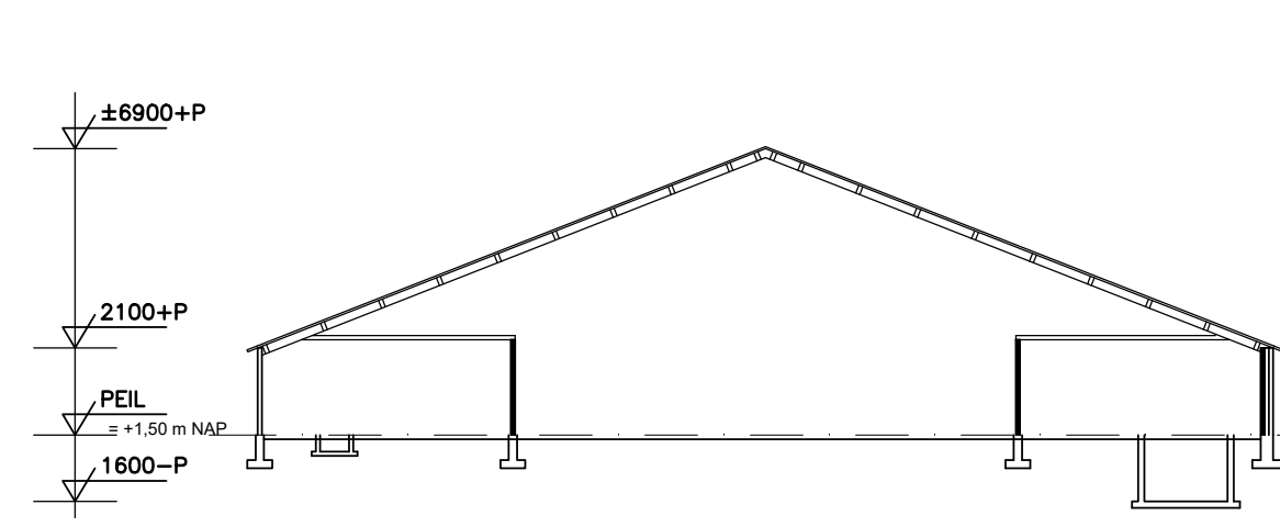
Doorsnede A-A
