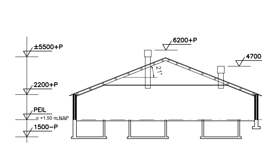
Doorsnede C-C
