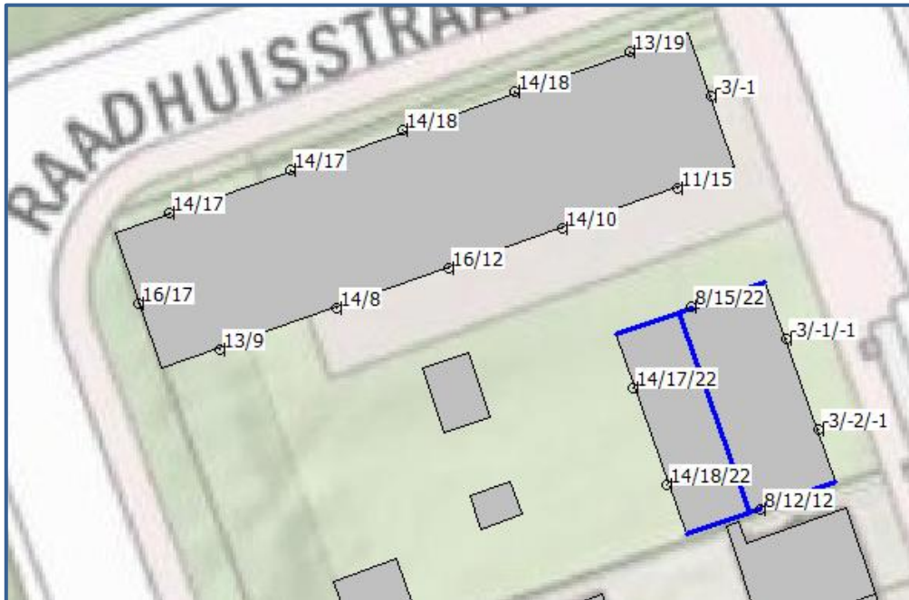
Afbeelding 8. Geluidbelastingen L_{den} (incl. aftrek art. 110g Wgh) Achterste Dijk Berekende geluidbelastingen op een hoogte van 1,5 / 4,5 / 7,5 meter
