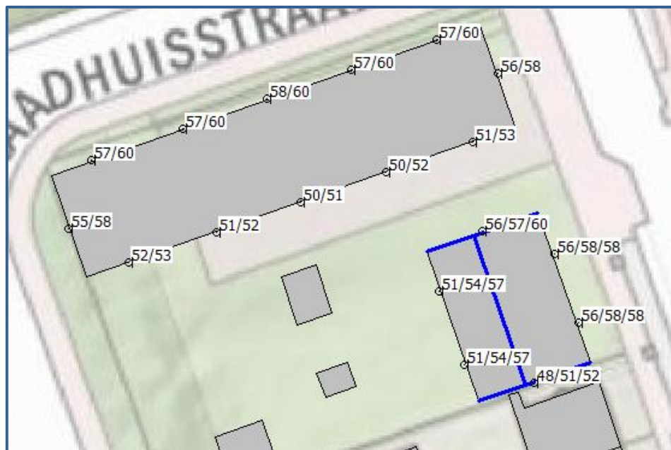
Afbeelding 10. Geluidbelastingen Lden (excl. aftrek art. 110g Wgh) cumulatief Berekende geluidbelastingen op een hoogte van 1,5 / 4,5 / 7,5 meter
