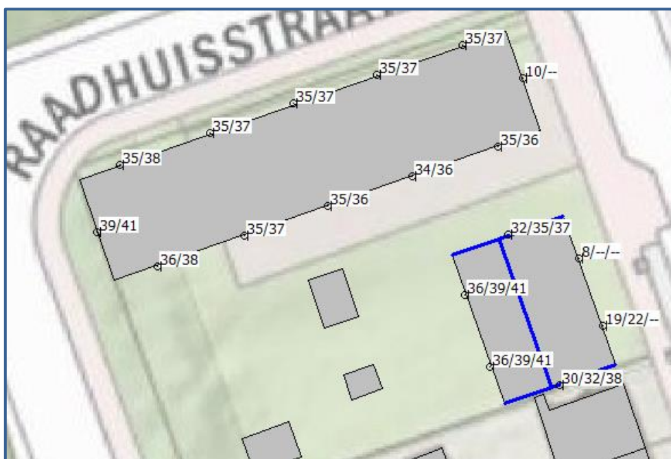
Afbeelding 7. Geluidbelastingen L_{den} (incl. aftrek art. 110g Wgh) Heemraadsingel Berekende geluidbelastingen op een hoogte van 1,5 / 4,5 / 7,5 meter
