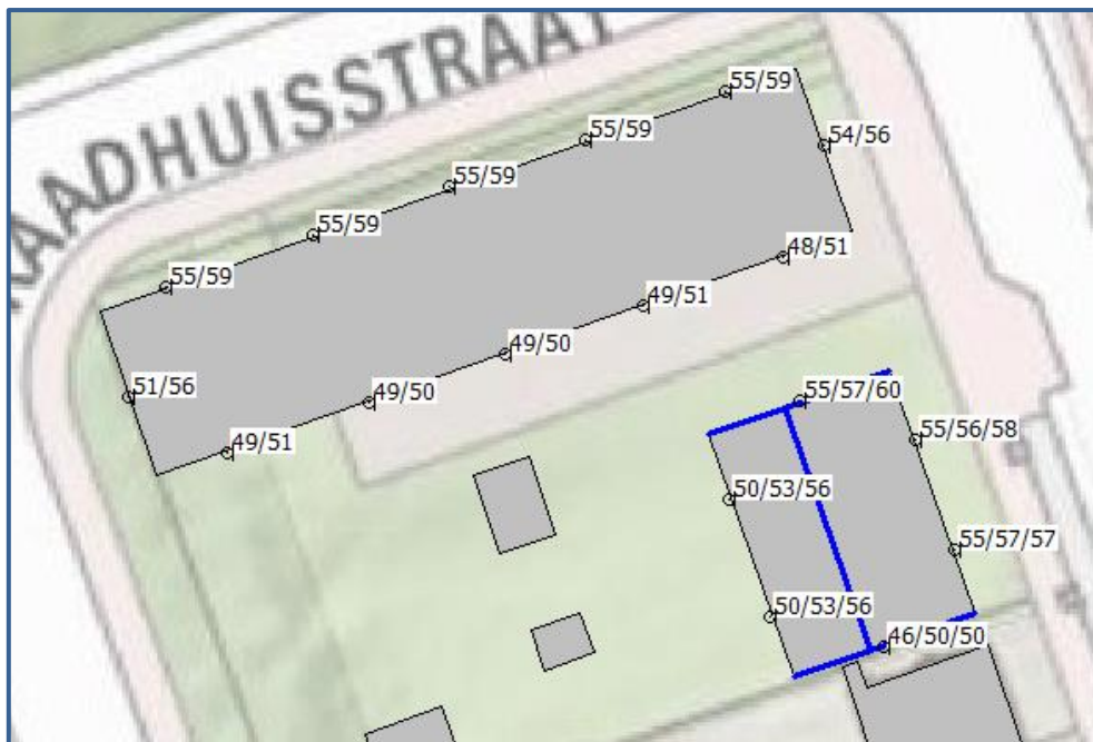
Afbeelding 9. Geluidbelastingen L_{den} (excl. aftrek art. 110g Wgh) A59 Berekende geluidbelastingen op een hoogte van 1,5 / 4,5 / 7,5 meter
