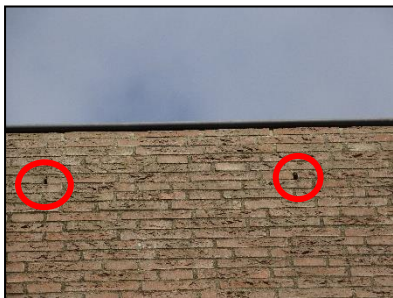
Figuur 13. Open stootvoegen (aangegeven met rode cirkels) van het kerkgebouw direct ten noorden van de onderzoekslocatie.
