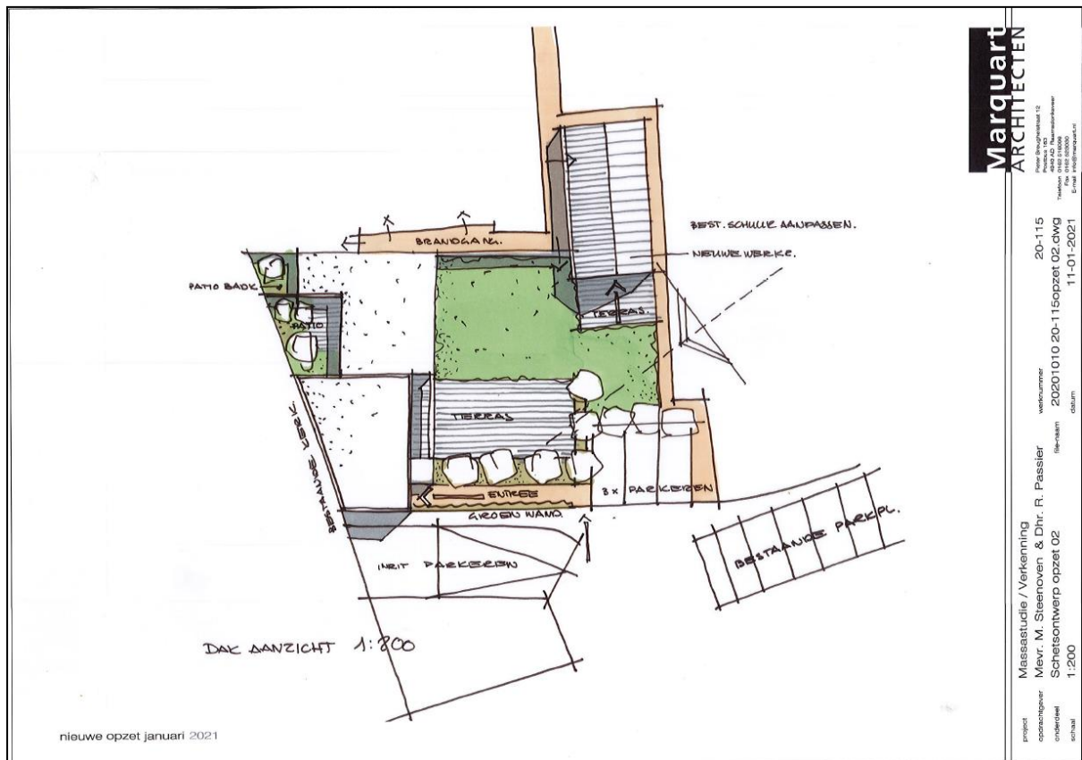
Figuur 9. Schetsontwerp van de nieuwbouw, de nieuwbouw is aangegeven met een wit gestippeld vlak. Bron: Marquart Architecten.
