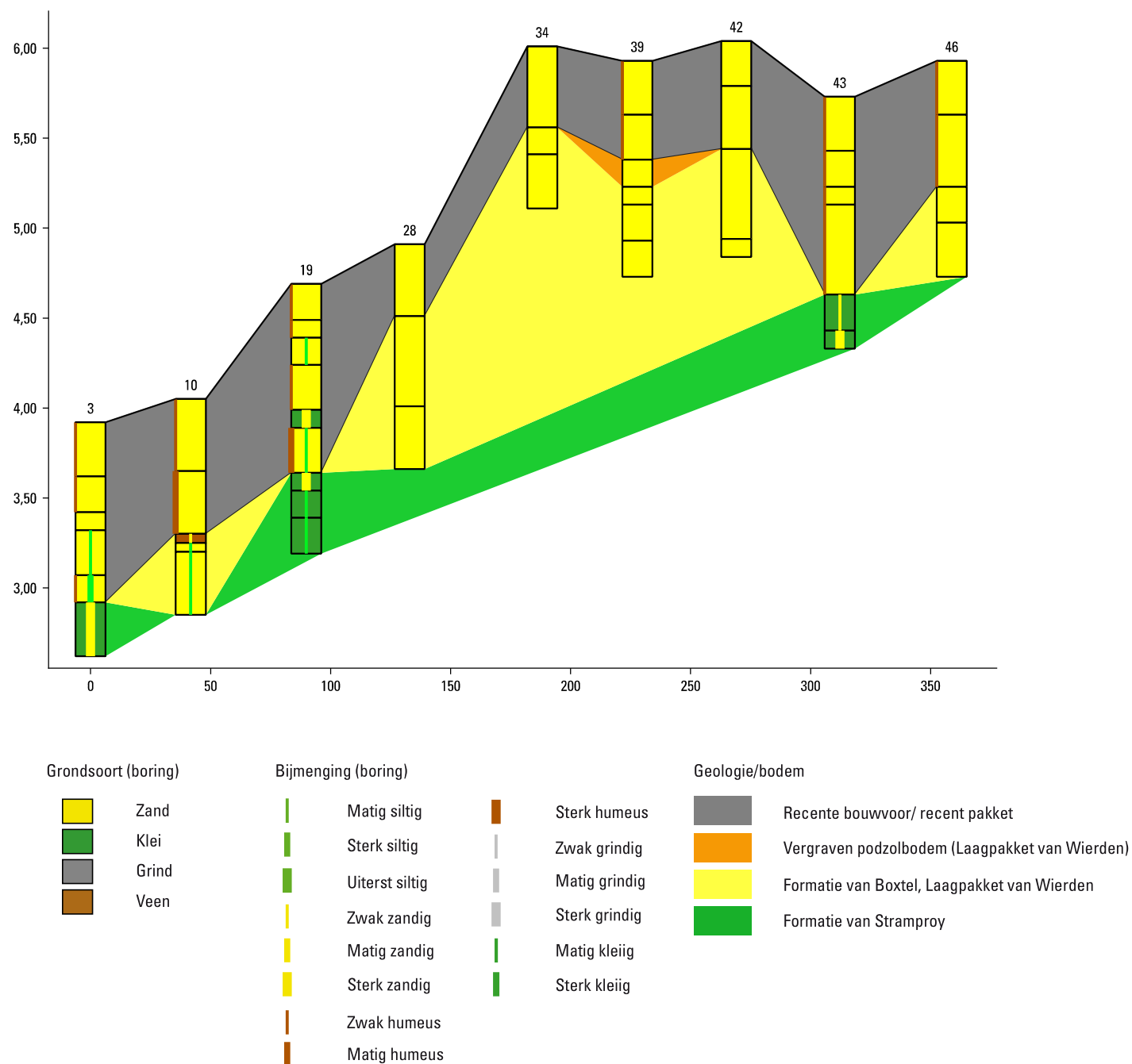
Bijlage 18a. Etten-Leur - Haansberg (deelgebied 3 tijdelijke woningen). Schematische doorsnede van het plangebied (Profiel A)
