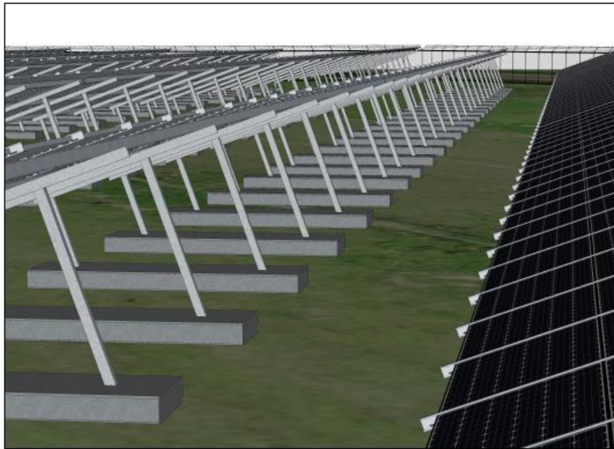
Opstelling in rijen - tussenruimte (indicatief)
