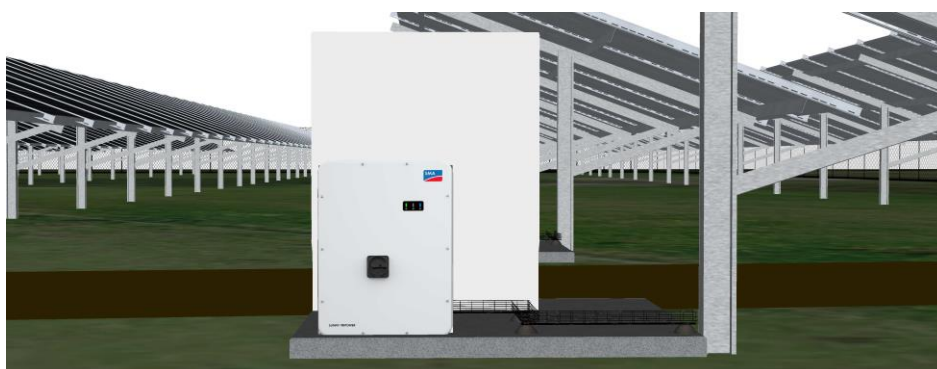
Voorbeeld plaatsing omvormers (aantal, mark en type nader te bepalen) (N.B.: getoonde draagconstructie wordt niet toegepast!)
