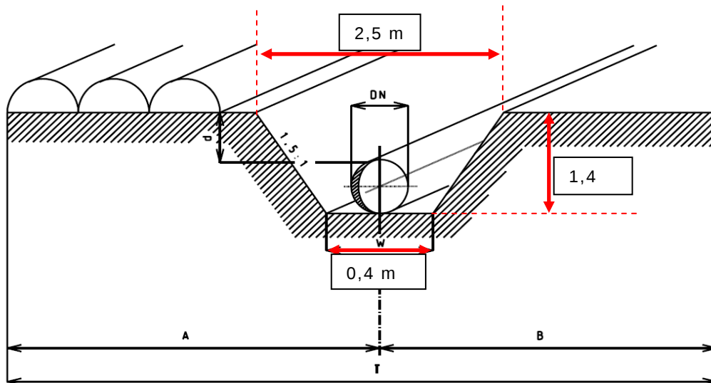
Figuur 3.2. Dwarsdoorsnede open ontgraving
