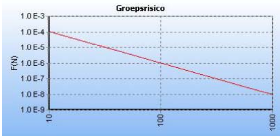
Figuur 3.4. Oriënterende waarde (rood) van het GR (fN-curve)
