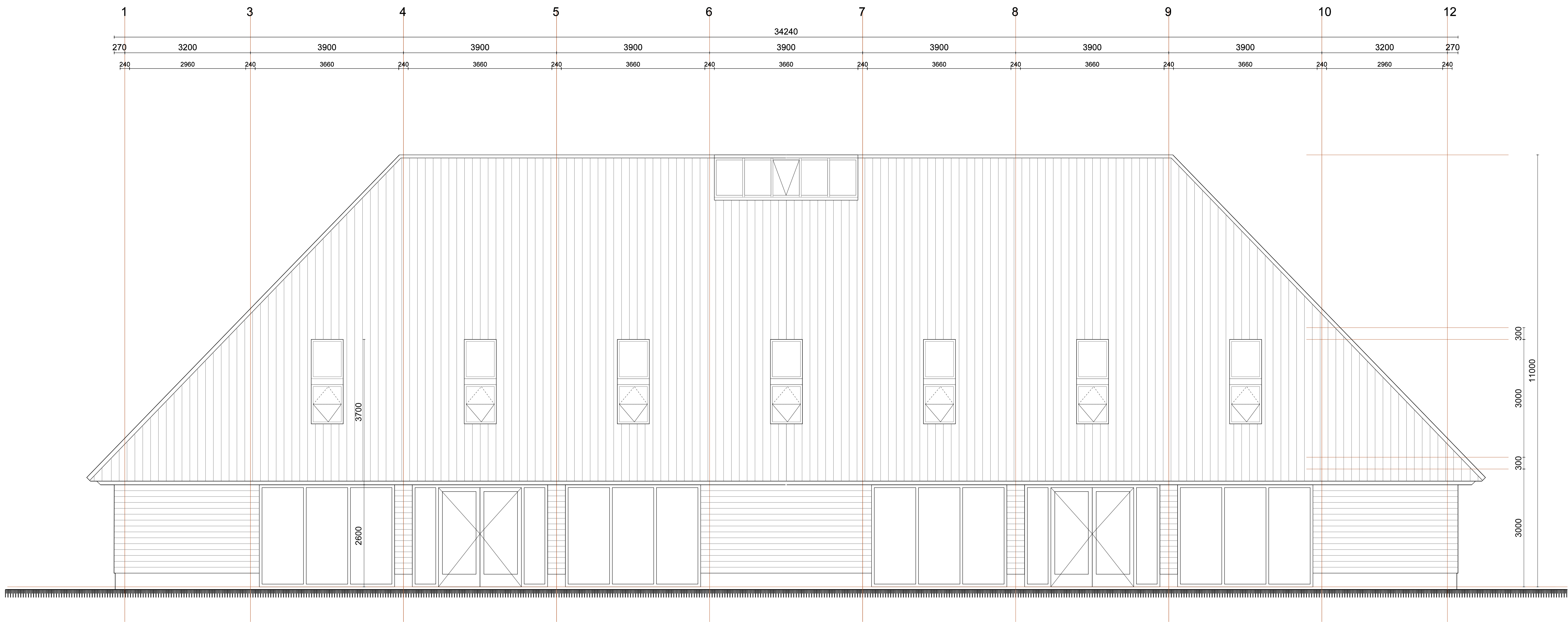
LANGSGEVEL NOORD-OOST
