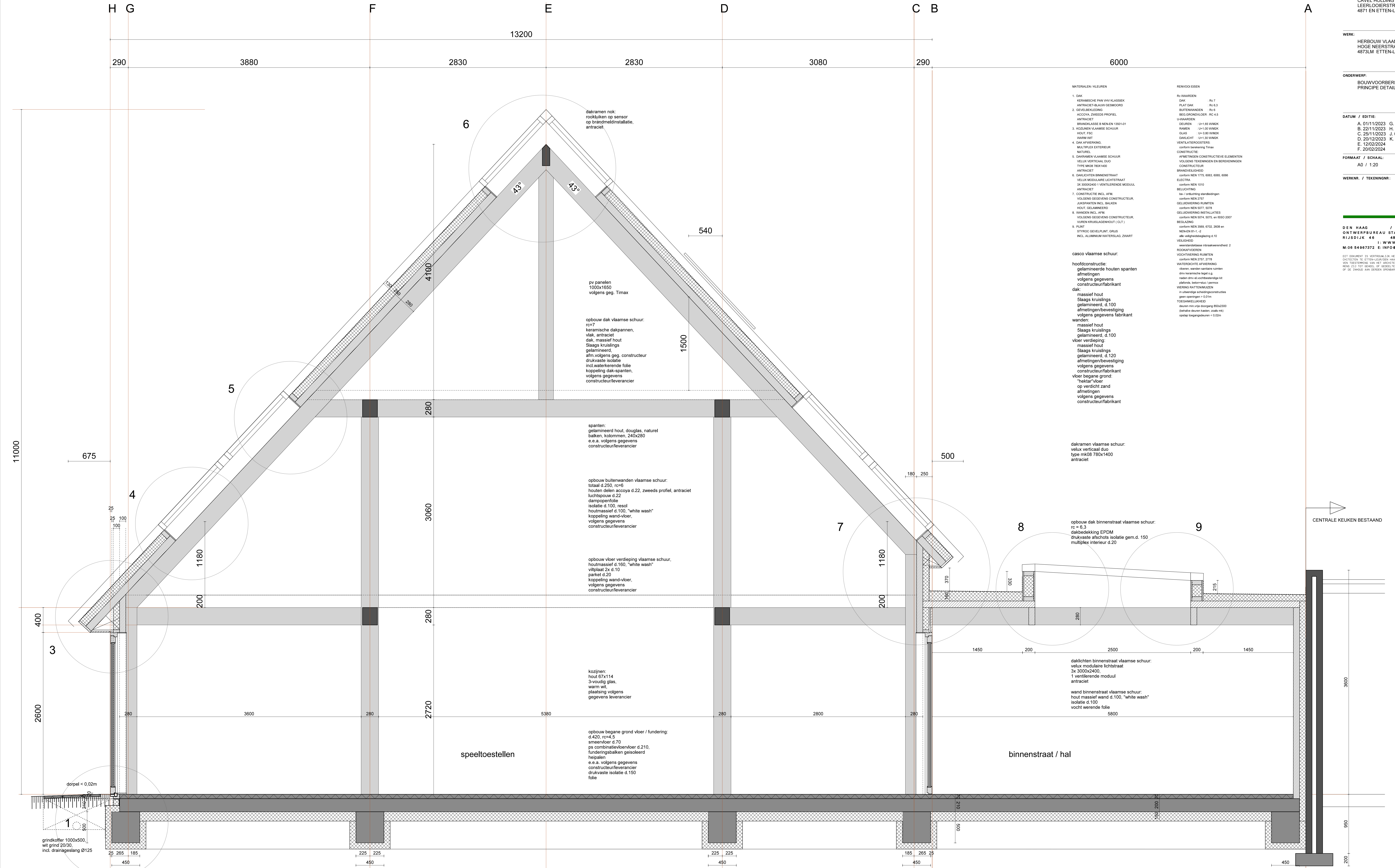
DETAIL DOORSNEDE A-A
