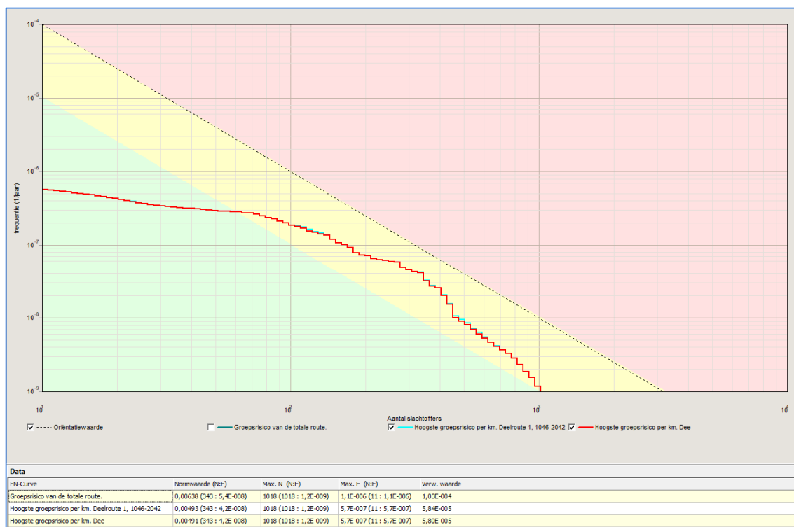
Afbeelding 6 fN-curves huidige situatie (rood) en beoogde situatie (blauw)
