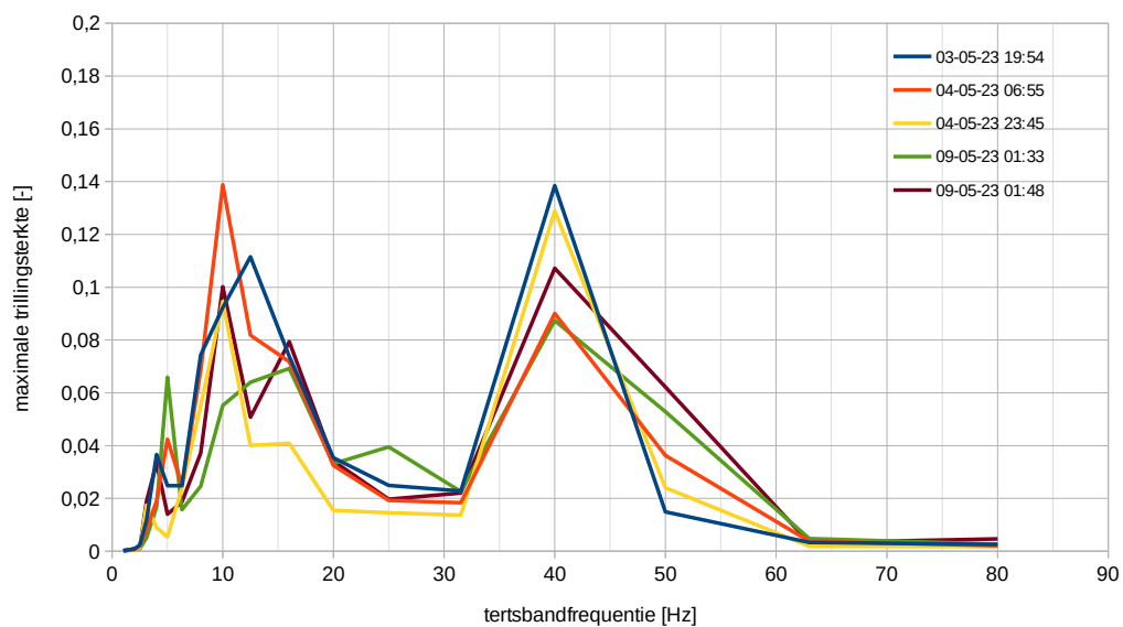
f2.2 Spectrale verdeling van de trillingsterkte als gevolg van de treinpassages (horizontale X richting)
