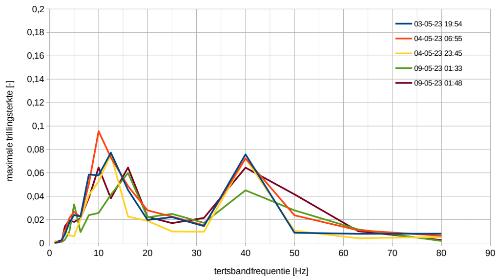
f2.3 Spectrale verdeling van de trillingsterkte als gevolg van de treinpassages (horizontale Y richting)
