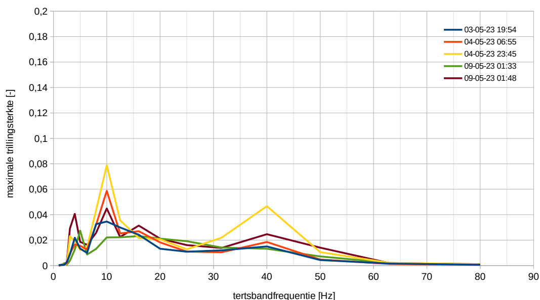
f2.4 Spectrale verdeling van de trillingsterkte als gevolg van de treinpassages (verticale Z richting)
