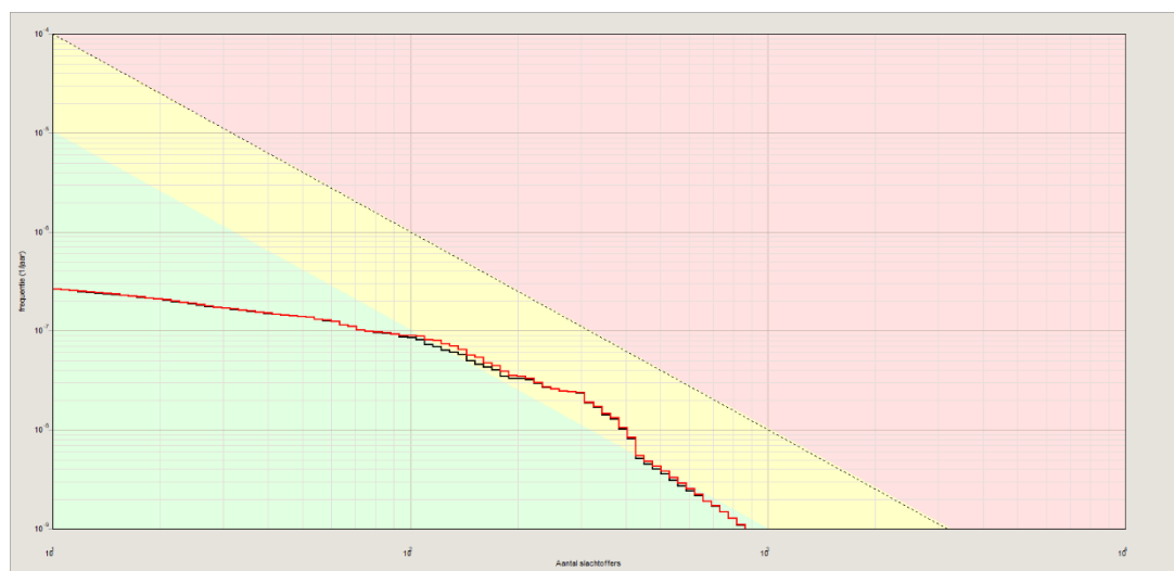
Figuur 3. Groepsrisicocurven
