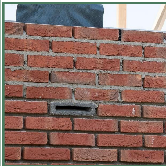
Ingebouwde vleermuiskast
