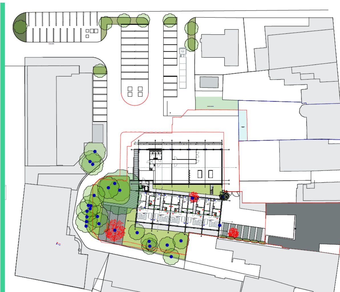
Afbeelding 2: ontwerptekening
