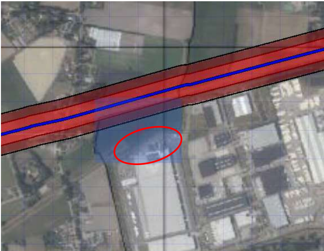
Abbeelding 2 Uitsnede CAROLA invloedsgebied buisleiding Z-520-37-deel-1
