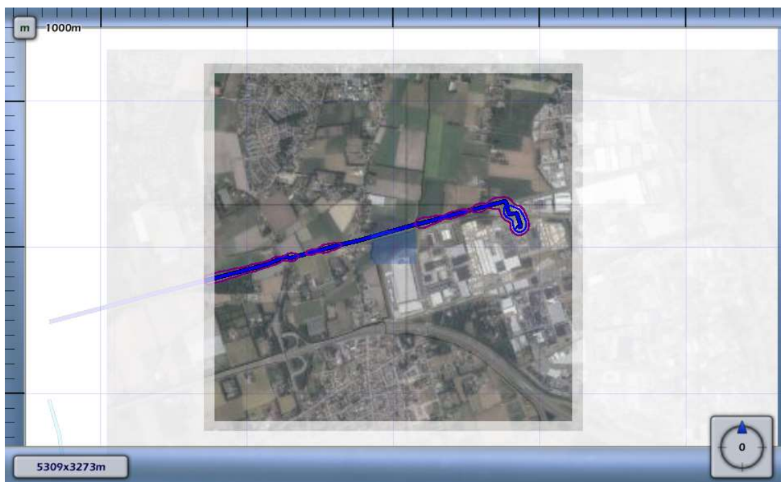
3.1 Figuur 3.1 Plaatsgebonden risico voor 7155_leiding-Z-520-37-deel-1 van N.V. Nederlandse Gasunie
