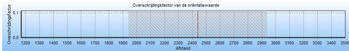
Afbeelding 6 Groepsrisico screening Z-520-37-deel-1, toekomstige situatie
