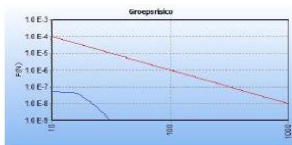
Figuur 4.4 FN-curve van de Z-539-01 in de toekomstige situatie
