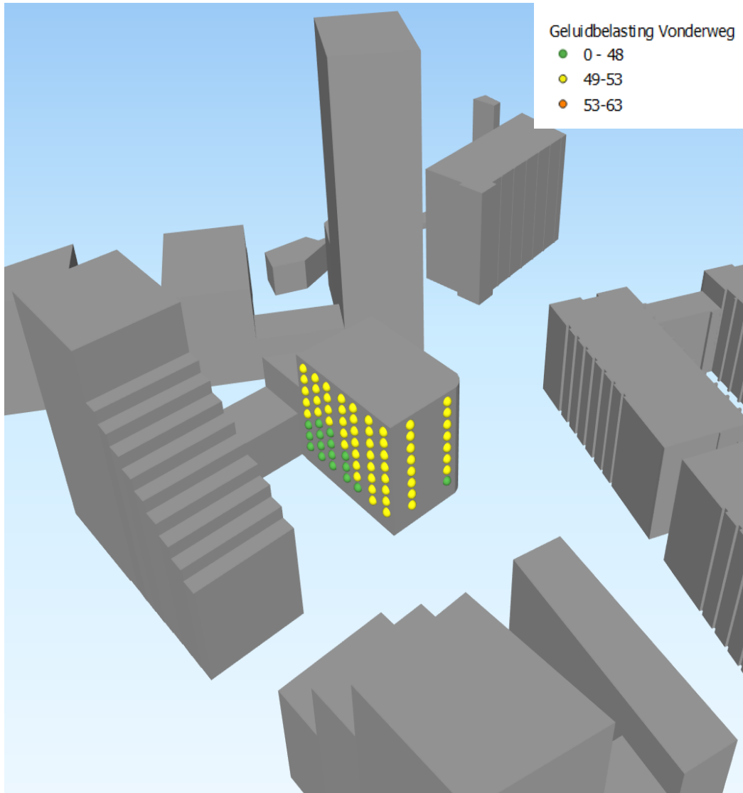
f3 Geluidbelasting ( L_{den} ) op Bouwblok C1 ten gevolge van de Vonderweg inclusief aftrek west- en zuidgevel
