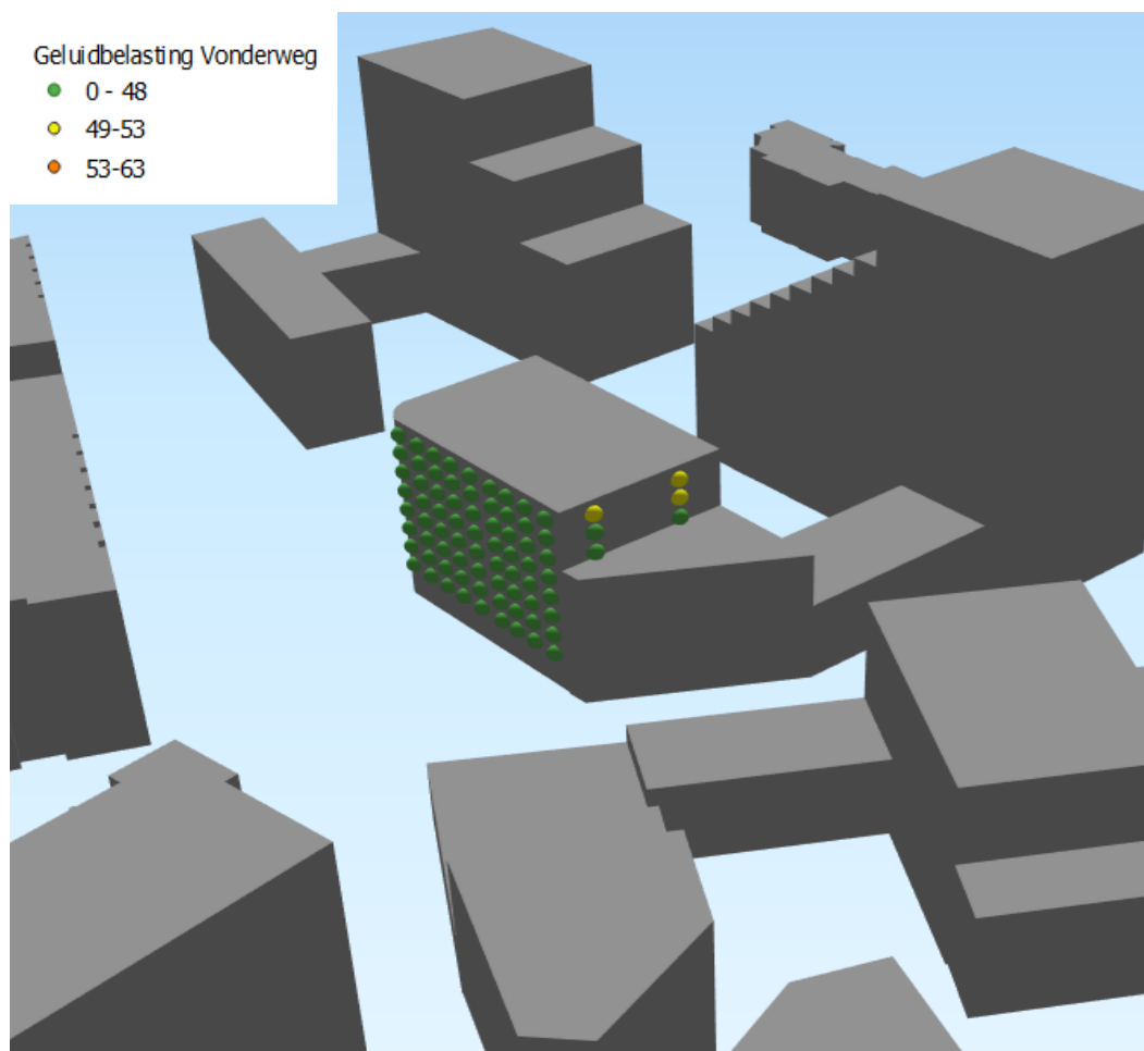
f4 Geluidbelasting ( L_{den} ) op Bouwblok C1 ten gevolge van de Vonderweg inclusief aftrek noord- en oostgevel
