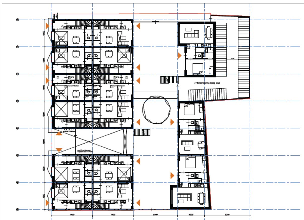
Figuur 1: Plattegrond van de begane grond in de toekomstige situatie.
