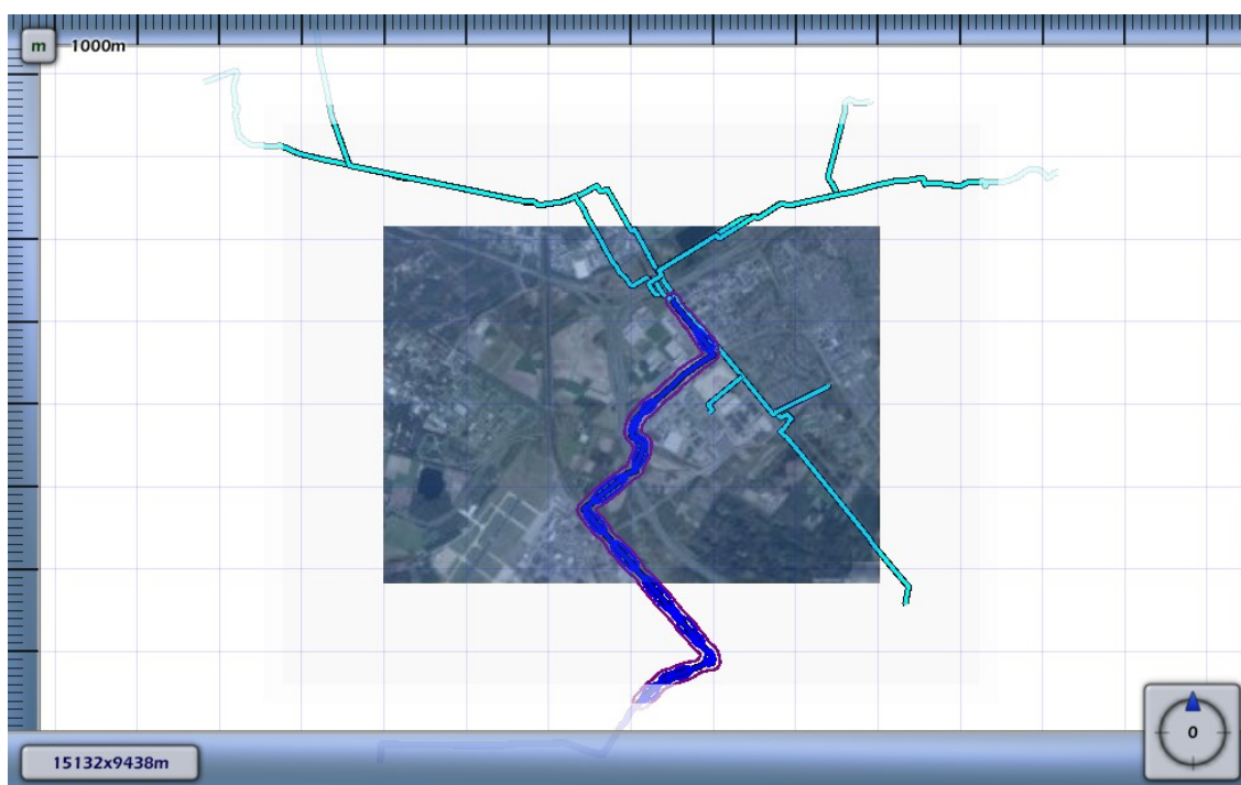
3.1 Figuur 3.1 Plaatsgebonden risico voor 5159_leiding-Z-506-01-deel-1 van N.V. Nederlandse Gasunie
