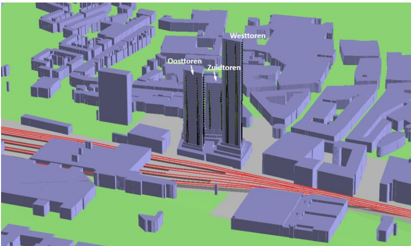
Figuur 6: 3D weergave rekenmodel railverkeer
