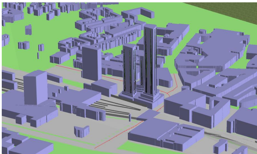
Figuur 7: 3D weergave rekenmodel railverkeer (bron: Geomilieu 4.41)
