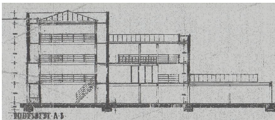
Afb. 38 Bouwtekeningen van het Van der Schootpand uit 1931.
