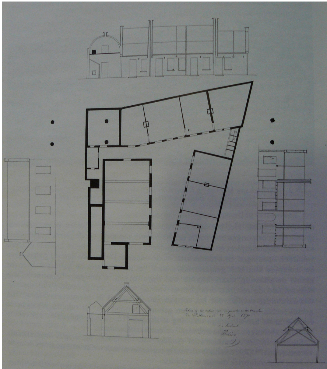
Afb. 18 Bouwtekening van de fabriek behorende bij het besluit van B & W d.d. 24 april 1870.
