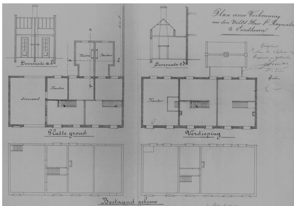
Afb. 27 Bouwtekening uit 1892.
