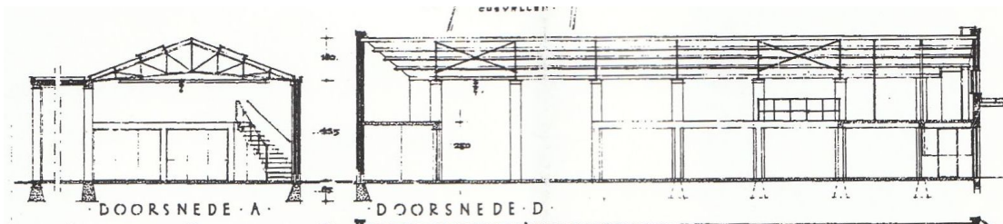
Afb. 40 Bouwtekening van de nieuwe loods behorend bij het pand Kleine Berg 45.
