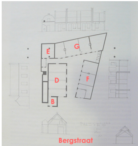
Afb. 24 Bouwtekening van de fabriek uit 1870, waarop de verschillende volumes in overeenstemming met de situatie op het briefhoofd zijn aangeduid.
