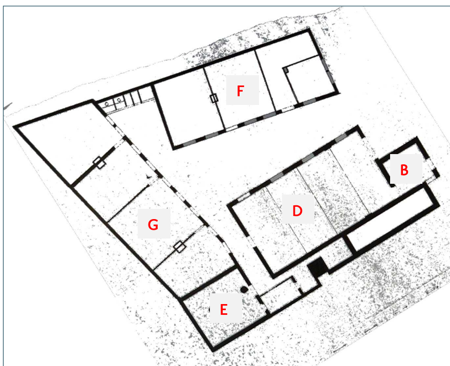
Afbeelding 2 Bouwtekening van de fabriek uit 1870 met daarbij de diverse ruimtes: B: Stoomwerktuig & Ketel; D: Zaag en schilmachines; E: Eest (droogkamer); F: bergruimte, kantoor en fabricage schoensmeer; G: dopen van de lucifers in witte fosfor. Bron: Pellemans & Rackham 2009.
