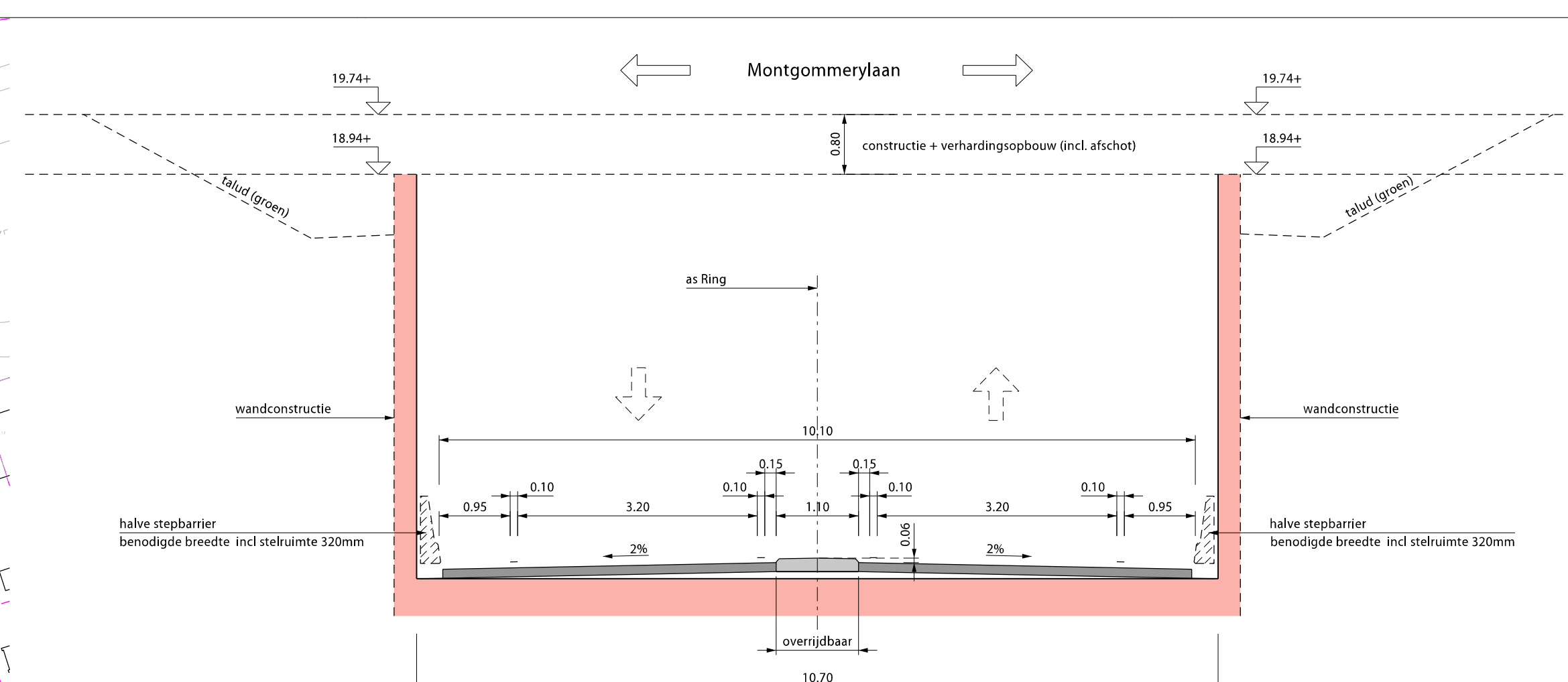
Dwarsprofiel A-A (Ring) Schaal 1:50
