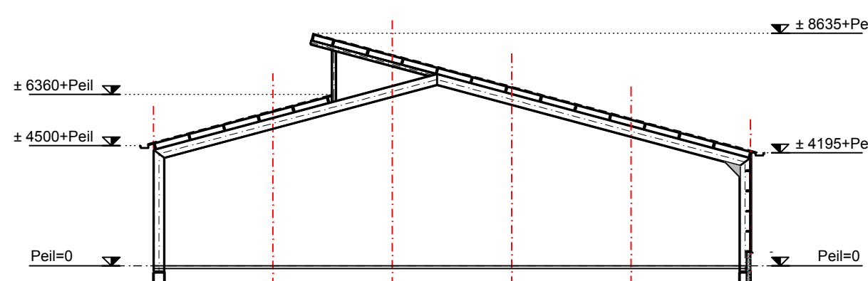
Doorsnede mestverwerker
