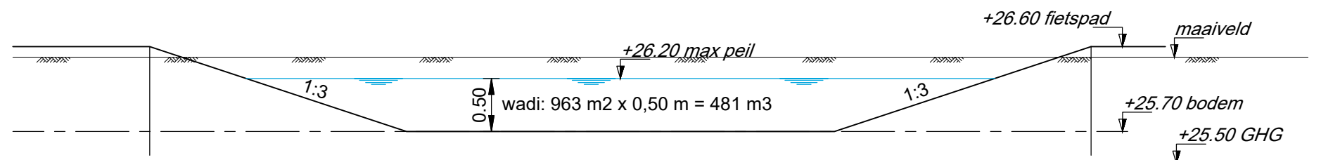
profiel A - A waterberging/ wadi 1:50
