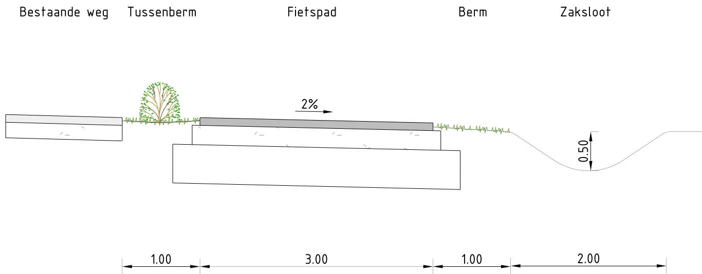
Principe profiel B-B Schaal 150
