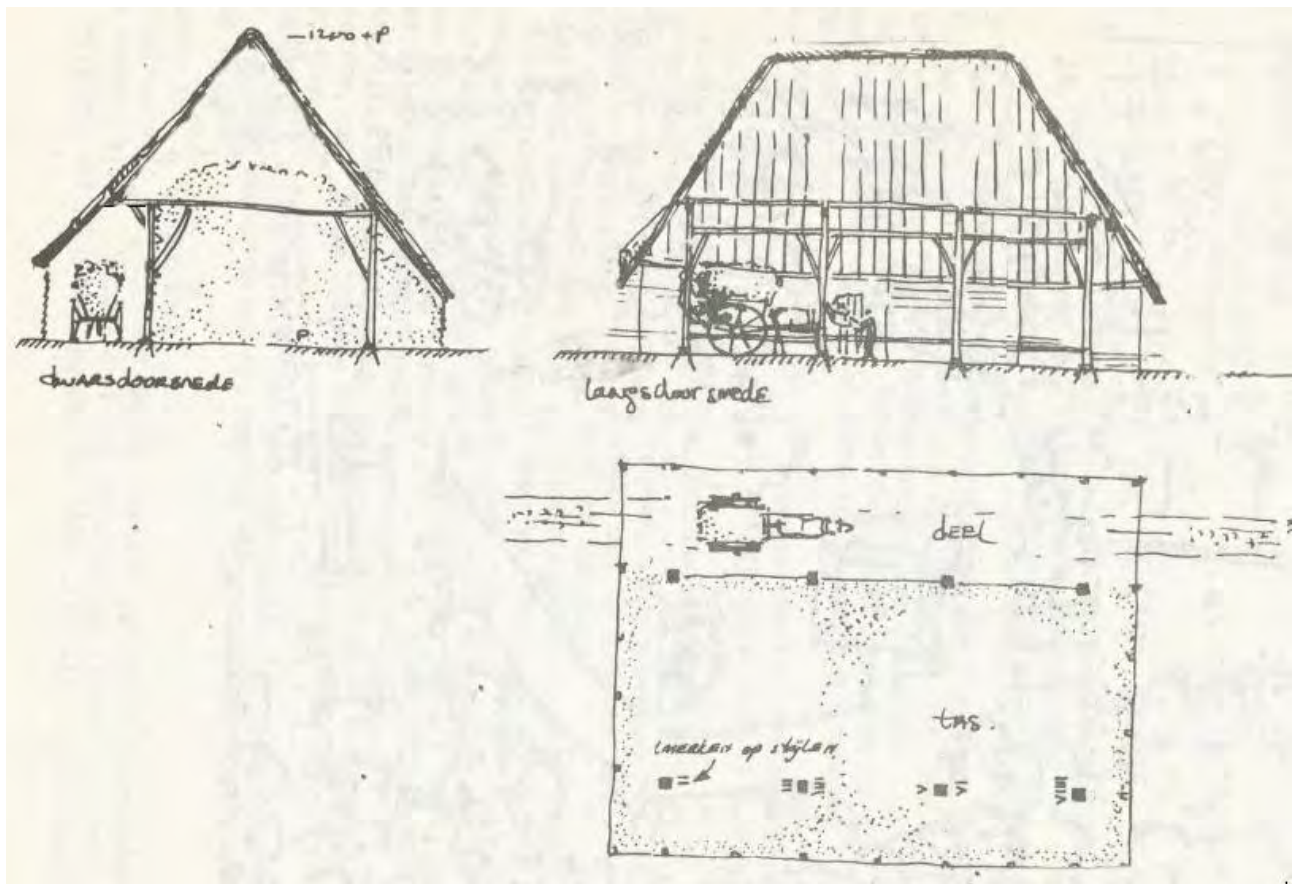
Principe van de Vlaamse schuur. Tekening uit 1971, digitaal aangepast om naar eigenschappen Groenstraat 9a.
