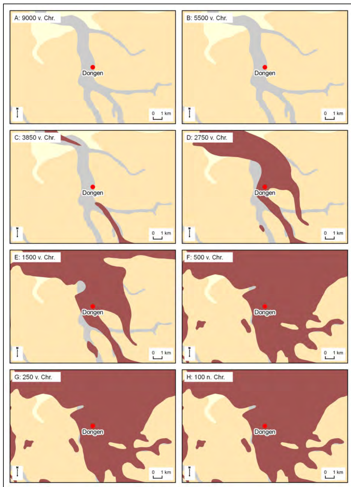
Figuur 5. Het plangebied op de paleogeografische kaart
