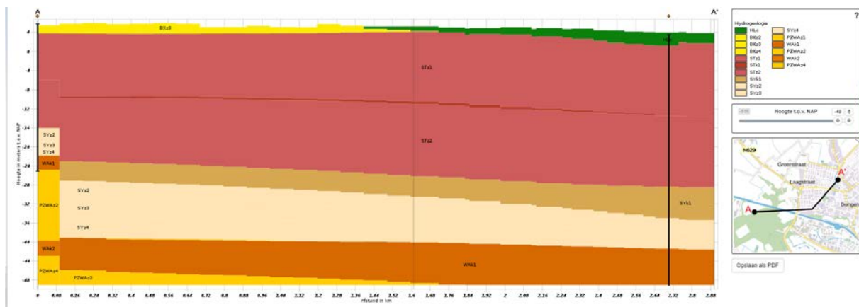
Figuur 2.1: Verticale doorsnede van de lithostratigrafie. De locatie ligt op 1,6 km vanaf punt A.
