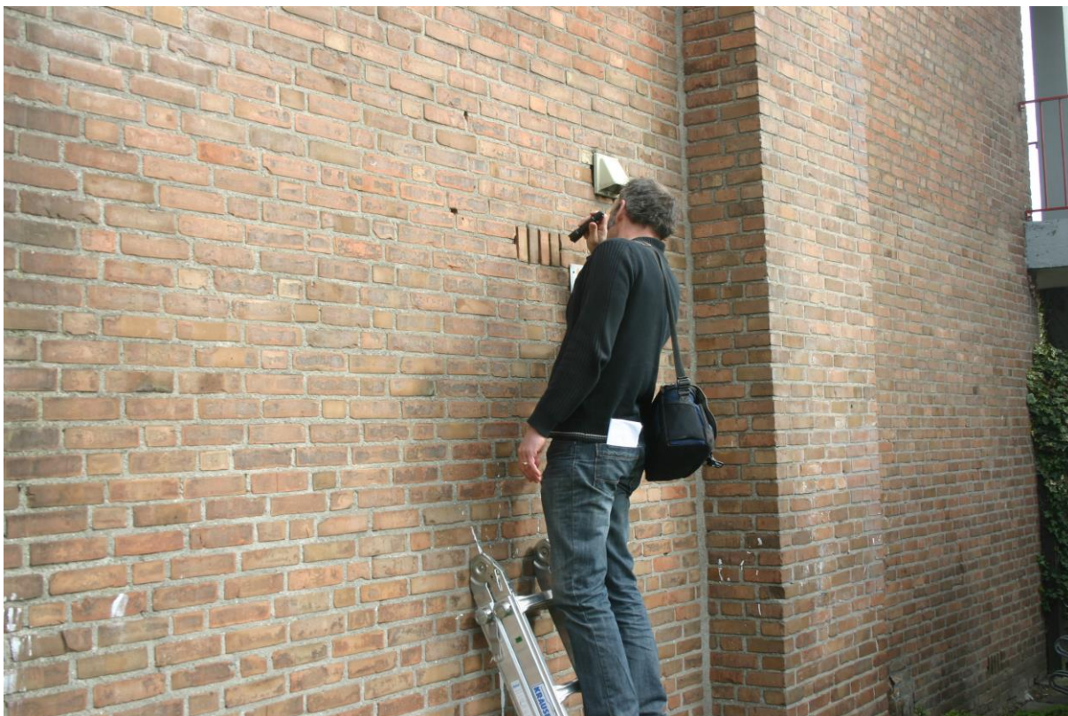
Figuur 2. Elke kopgevel aan de zuidzijde bevat 5 naast elkaar gelegen open stootvoegen.
