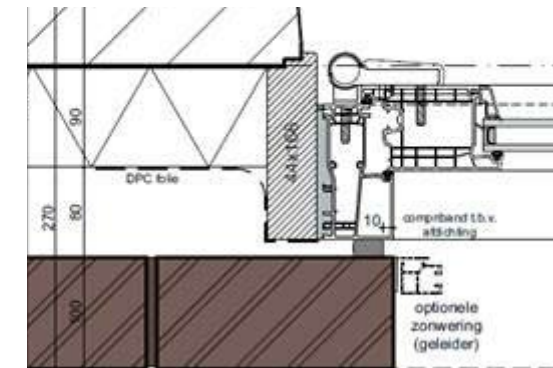
principedetail kozijnen
