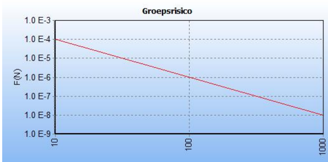
Figuur 8 FN-curve van gastransportleiding N-523-83 in de toekomstige situatie.
