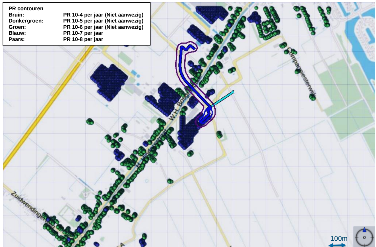
Figuur 4 PR contouren en ligging van de gastransportleiding N-523-83 (donkerblauw) in de toekomstige situatie
