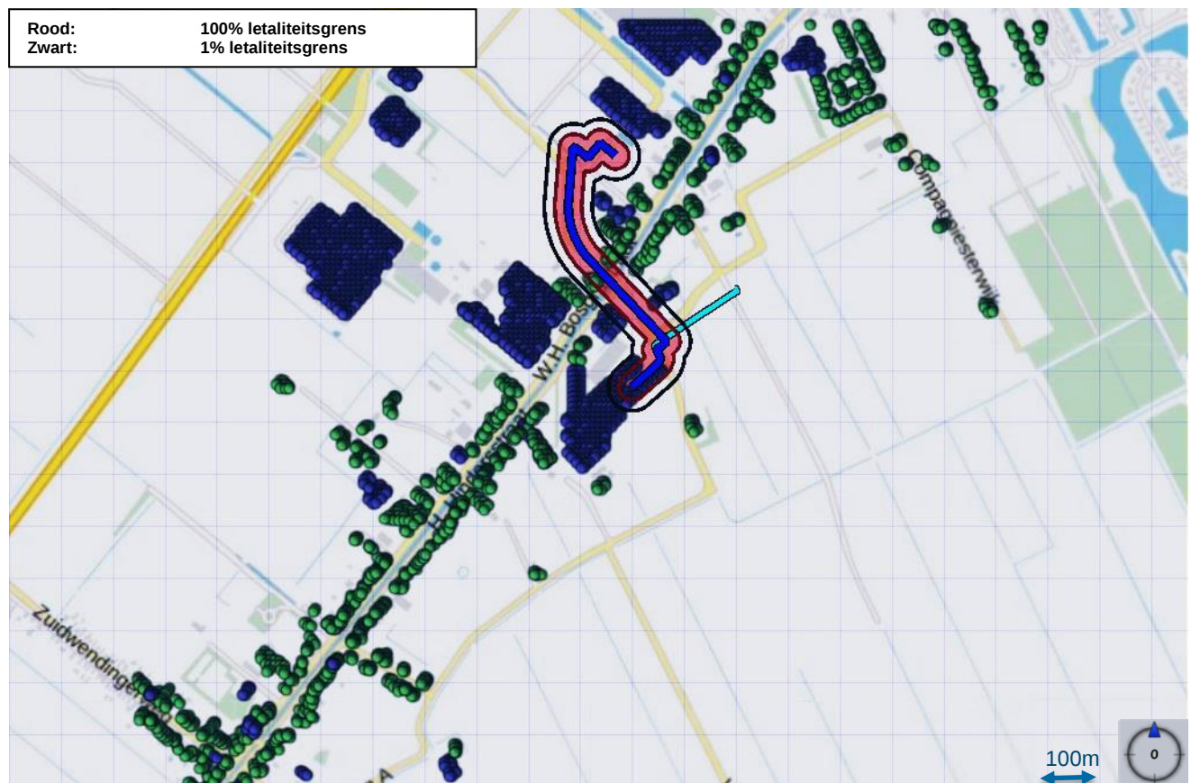
Figuur 2 Invloedsgebied van de leiding N-523-83 (donkerblauw) in de toekomstige situatie.
