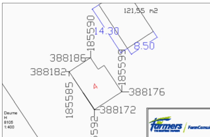
Figuur 1: Coördinaten hoekpunten bedrijfswoning.
