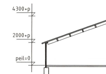
Doorsnede B-B
