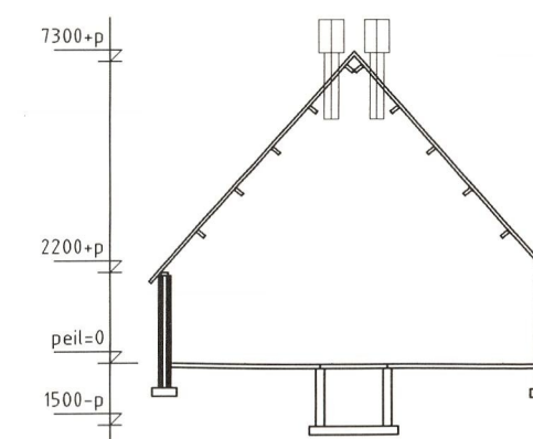
Doorsnede A-A
