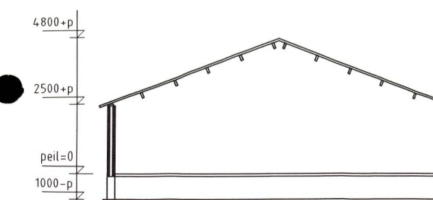
Doorsnede D-D
