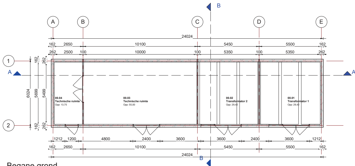
Begane grond
