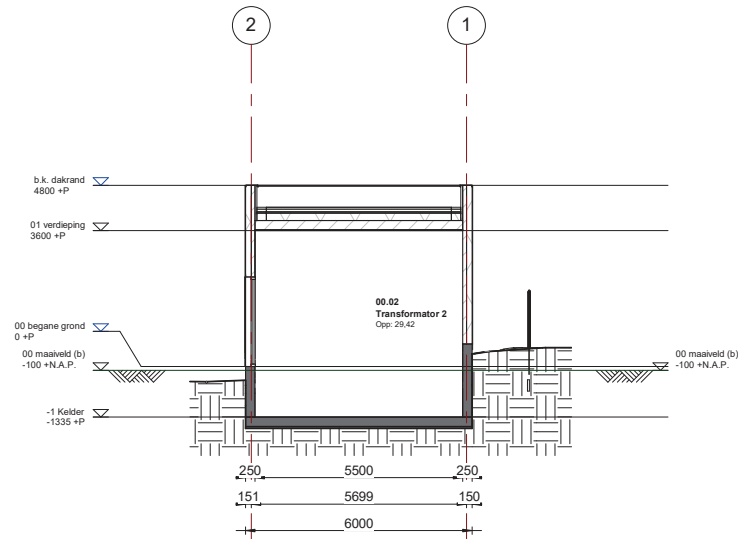
Doorsnede B-B
