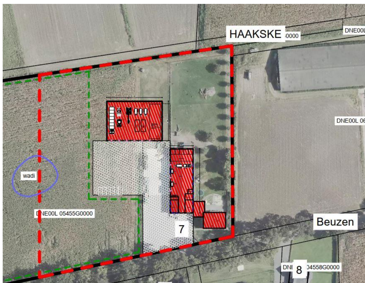
Afbeelding 7: bestaande gecombineerd met nieuwe situatie na bouw loods en aanleg erfverharding.
