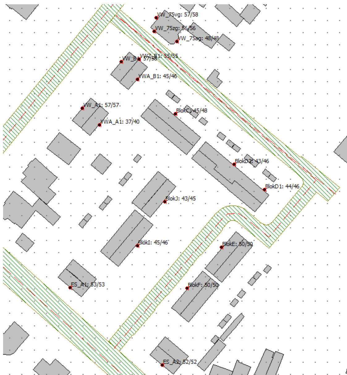
Afbeelding 4.4.1. Cumulatieve geluidbelastingen L_{den} [dB] op de beschouwde beoordelingshoogten (1,5/4,5 m)
