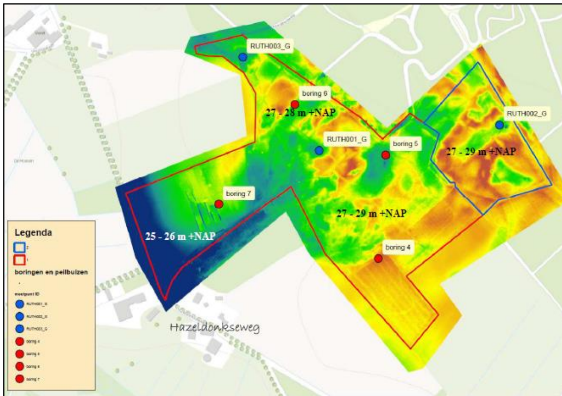
Afbeelding variatie maaiveldhoogten (bron: Geohydrologisch onderzoek; Landslide).
