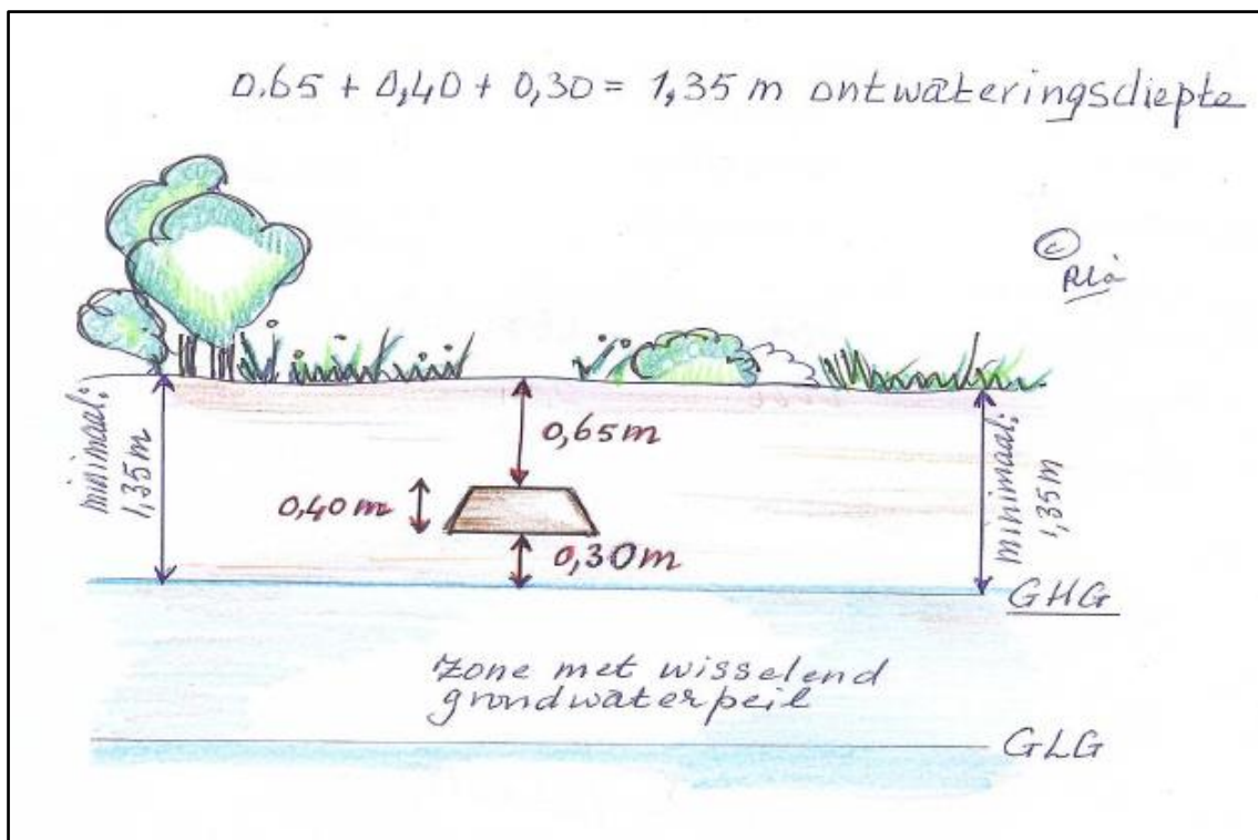
Afb. schematische weergave (dwarsdoorsnede) benodigde ontwateringsdiepte voor begraven.
