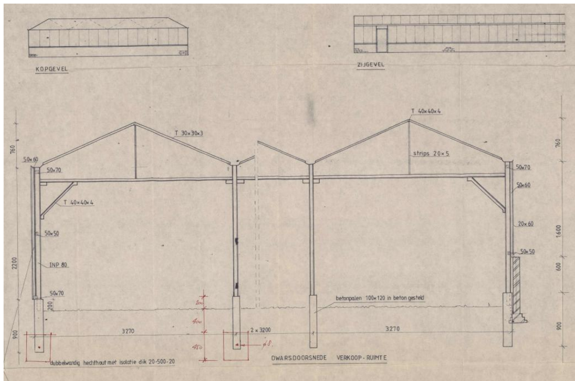
Afb. 3 Uitsnede van de bouwtekening van een deel van de kassen aan de Tilburgseweg.
