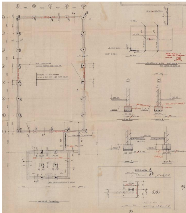
Afb. 4 Uitsnede van de bouwtekening van Aardenhoek 36-38.
