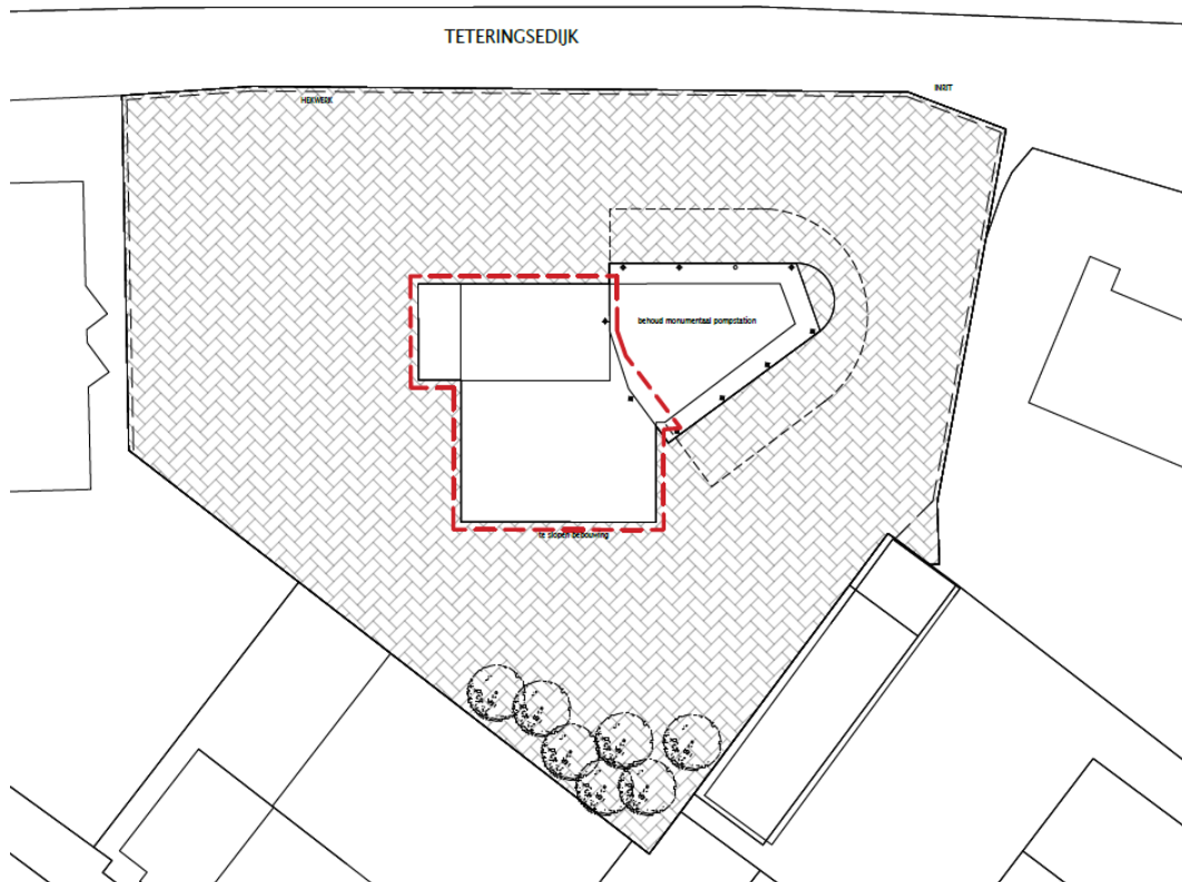
Figuur 1.3. Te slopen (rode contour) en te behouden deel van de bebouwing in het plangebied (BNArchitecten, 2021).
