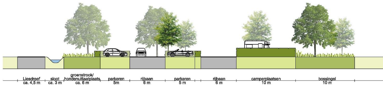
Figuur 6: Principendoorsnede A-A'
