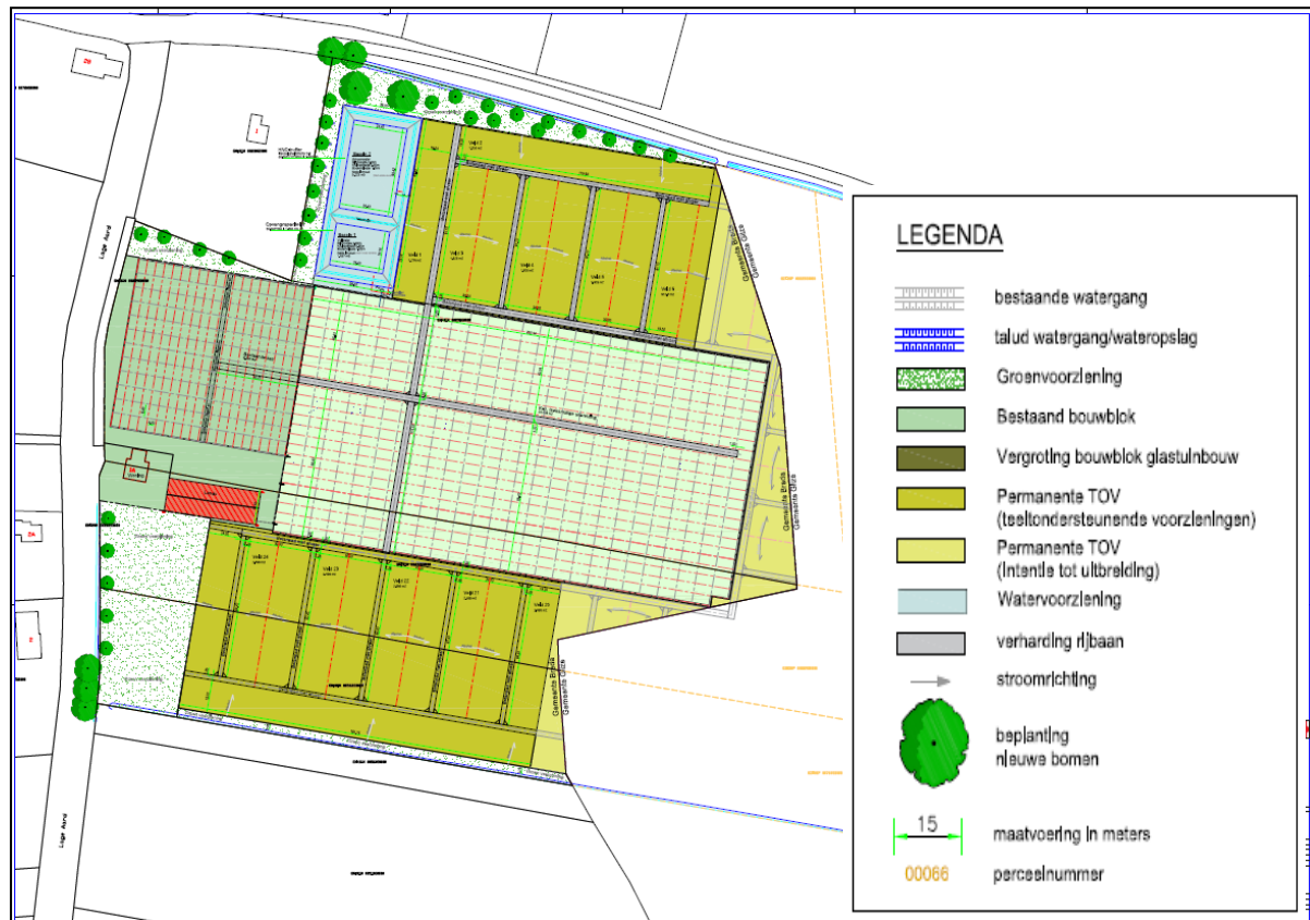
Figuur 9. Uitsnede inrichtingsplan (Bron: Traycon infra meting B.V.).
