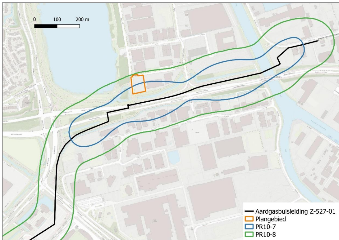
Figuur 3. Plaatsgebonden risicocontouren aardgasleiding Z-527-01
