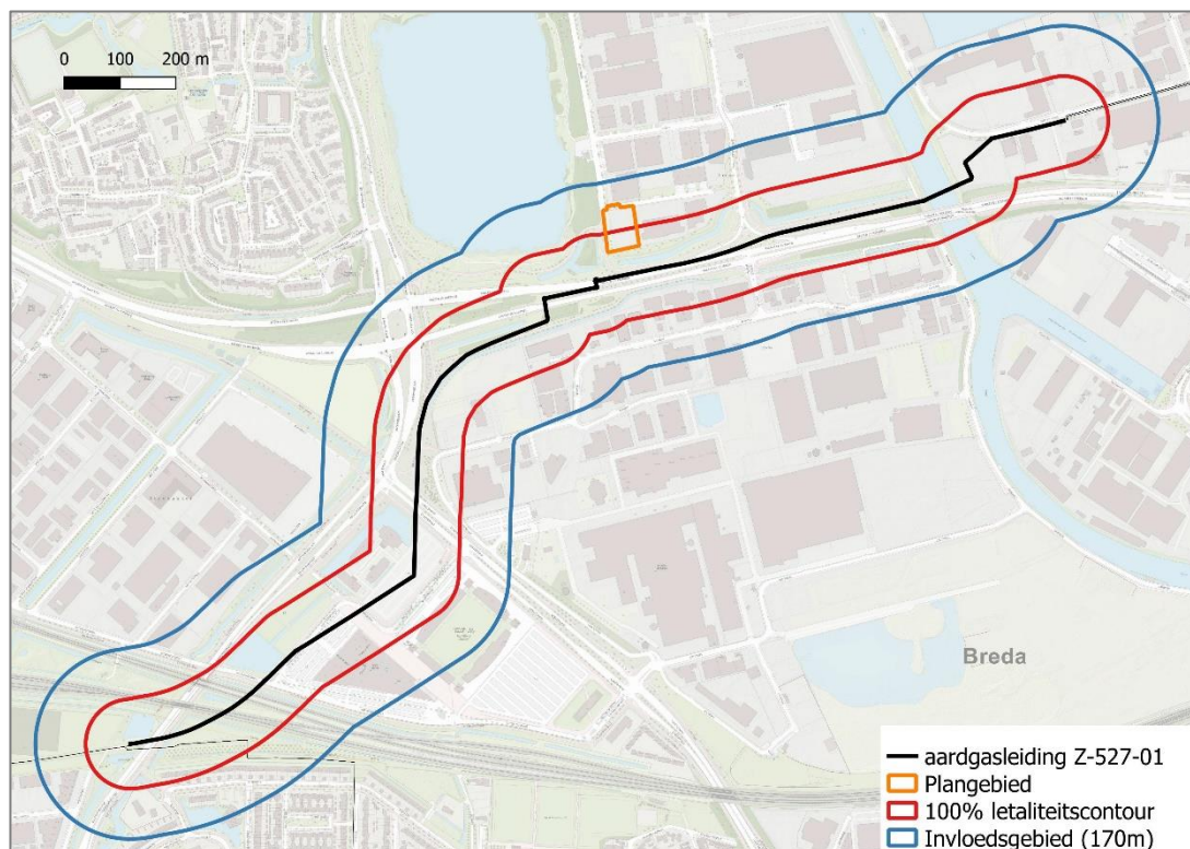
Figuur 2. Invloedsgebied (1% letaliteitszone) en 100%-letaliteitszone
