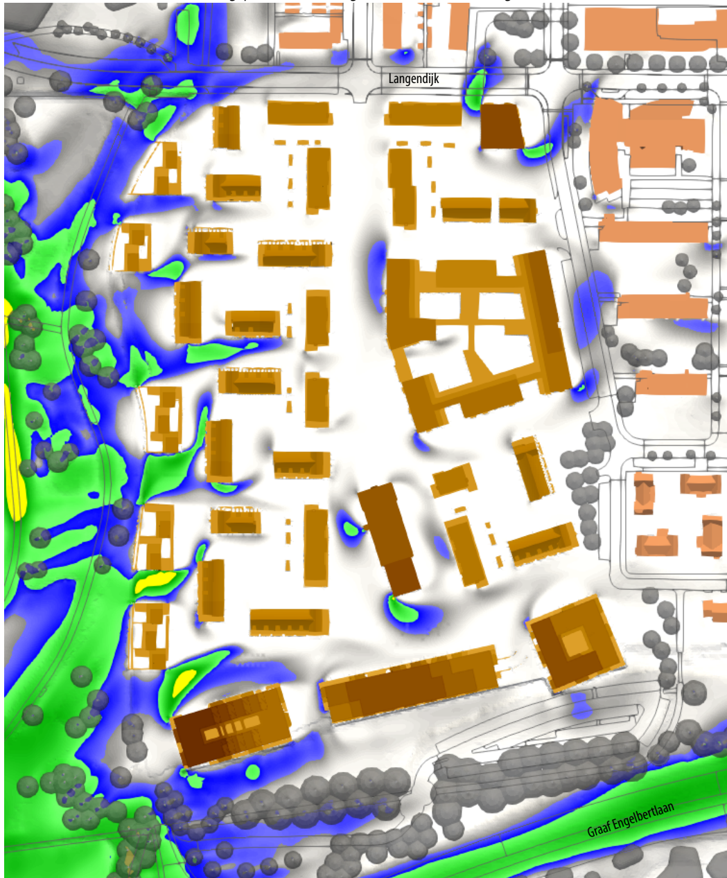
f3.2 Het te verwachten windklimaat in de geplande bebouwingssituatie, beoordeeld volgens de NEN 8100
