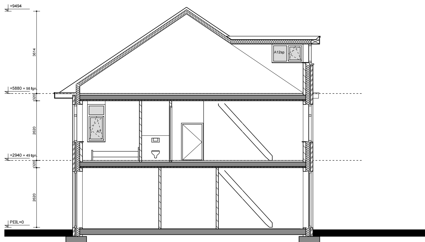
Doorsnede AA
