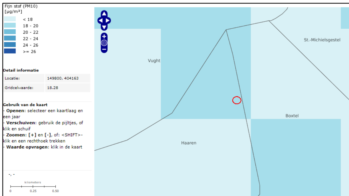
Afbeelding 17: Uitsnede GCN-Kaart PM_{10} , projectgebied met rood aangegeven.
