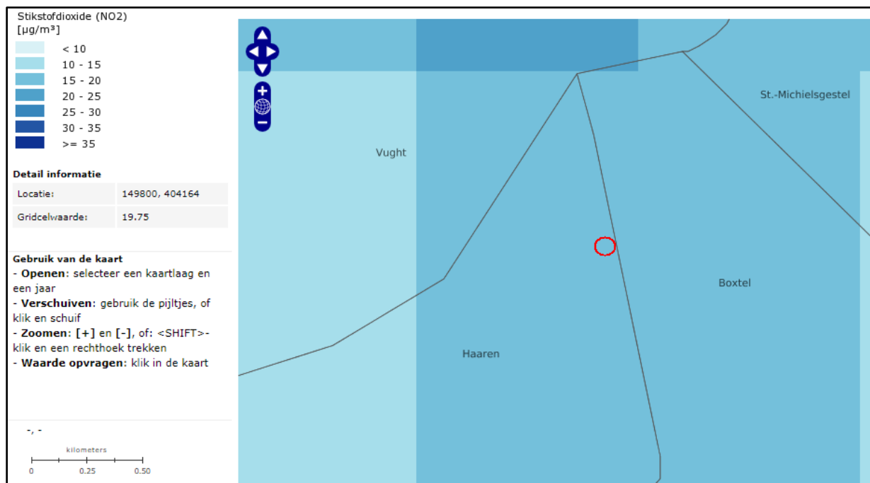
Afbeelding 19: Uitsnede GCN-Kaart NO 2 , plangebied met rood aangegeven.
