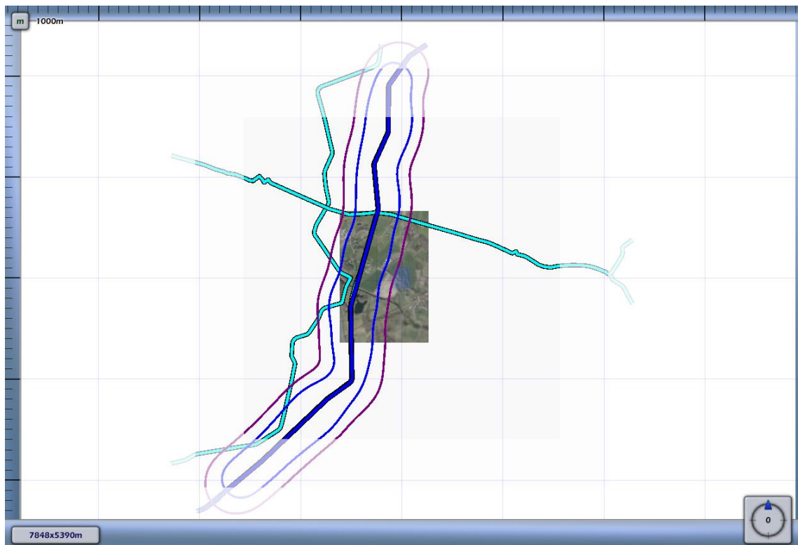
3.1 Figuur 3.1 Plaatsgebonden risico voor 8195_leiding-A-525-deel-1 van N.V. Nederlandse Gasunie
