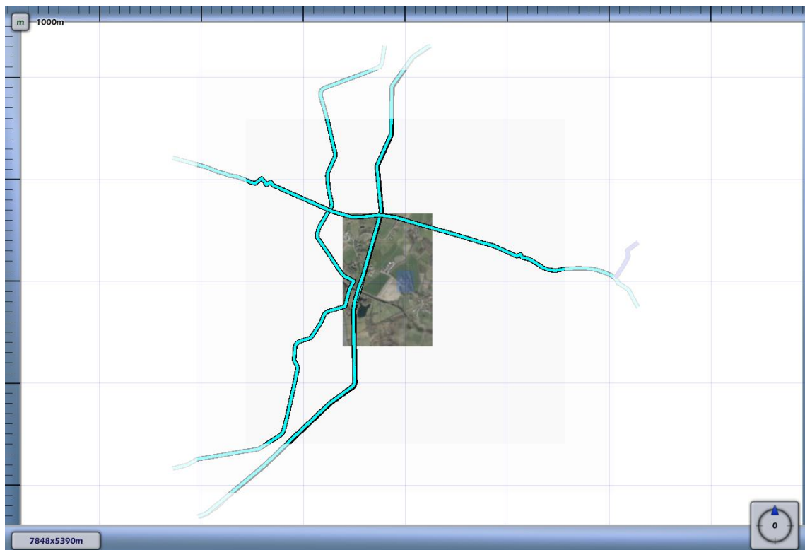
3.5 Figuur 3.5 Plaatsgebonden risico voor 8195_leiding-Z-544-03-deel-1 van N.V. Nederlandse Gasunie
