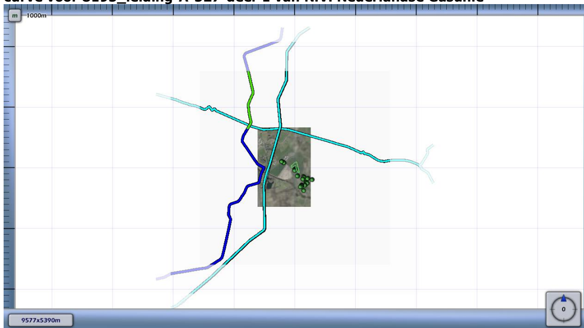
Figuur 4.3 Kilometer leiding behorende bij de maximale overschrijding van de FN-curve voor 8195_leiding-A-527-deel-1 van N.V. Nederlandse Gasunie
