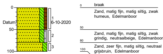
Inspectiegat/Boring: A06
