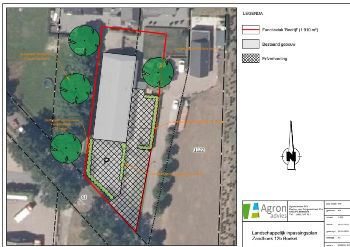
Figuur 131 Inrichtingsschets Zandhoek 12b
