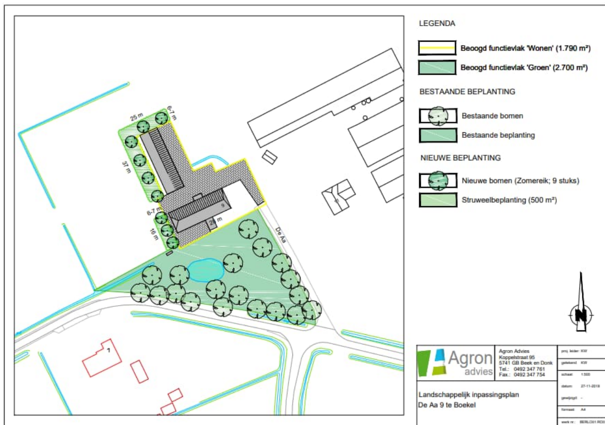
Figuur 86 Inrichtingsschets De Aa 9
