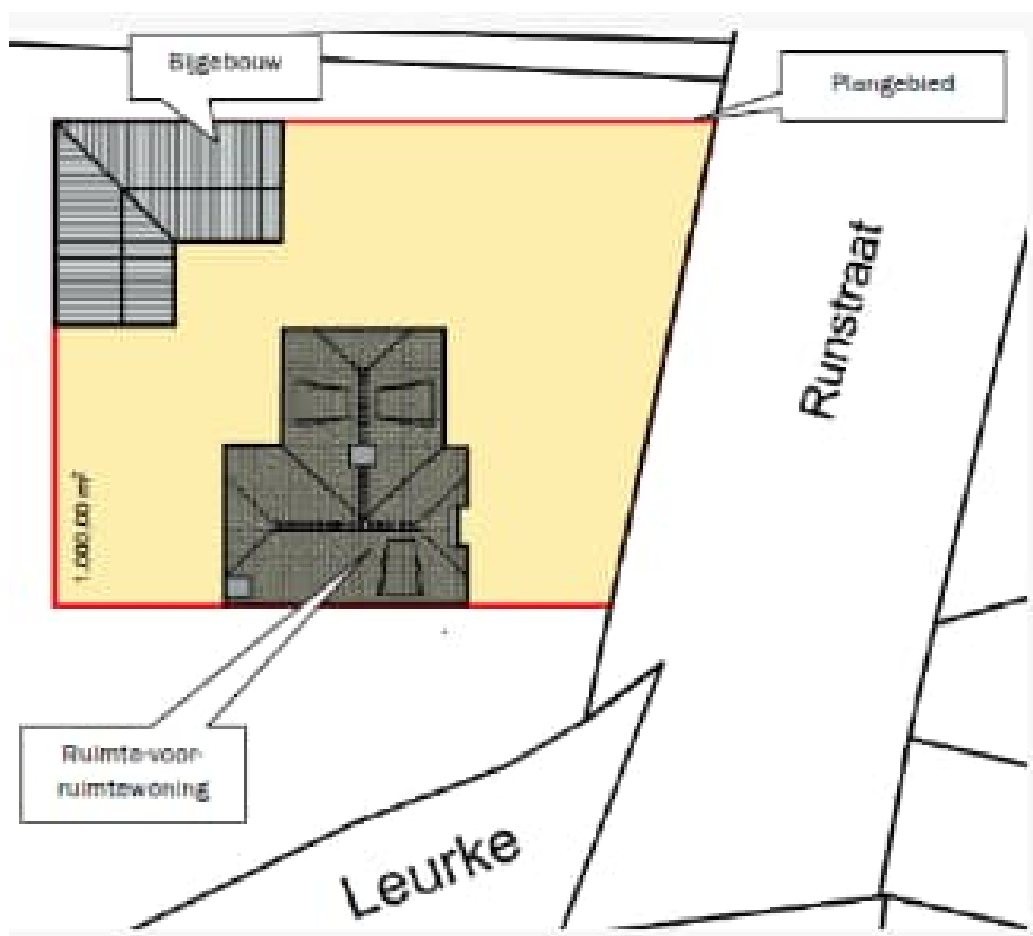
Figuur 63 Toekomstige Situatie
