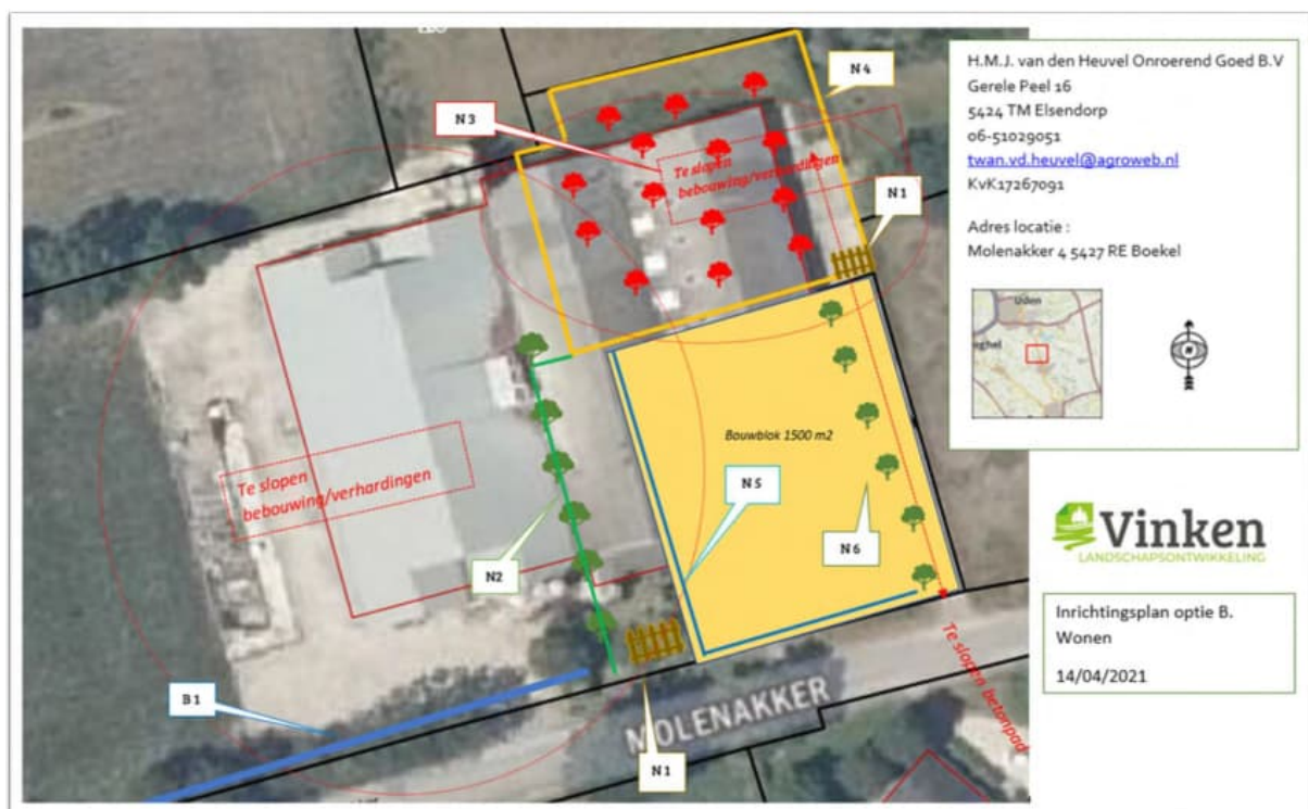
Figuur 145 Inrichtingsschets Molenakker 4
